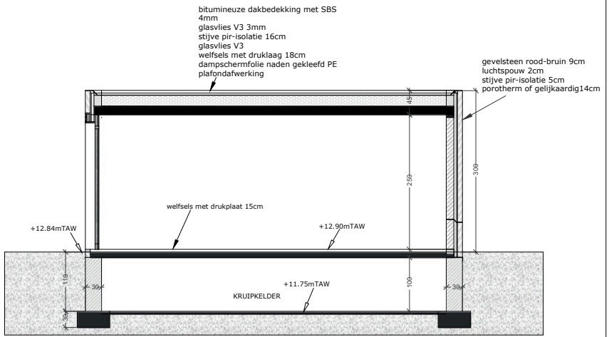
SNEDE BB
