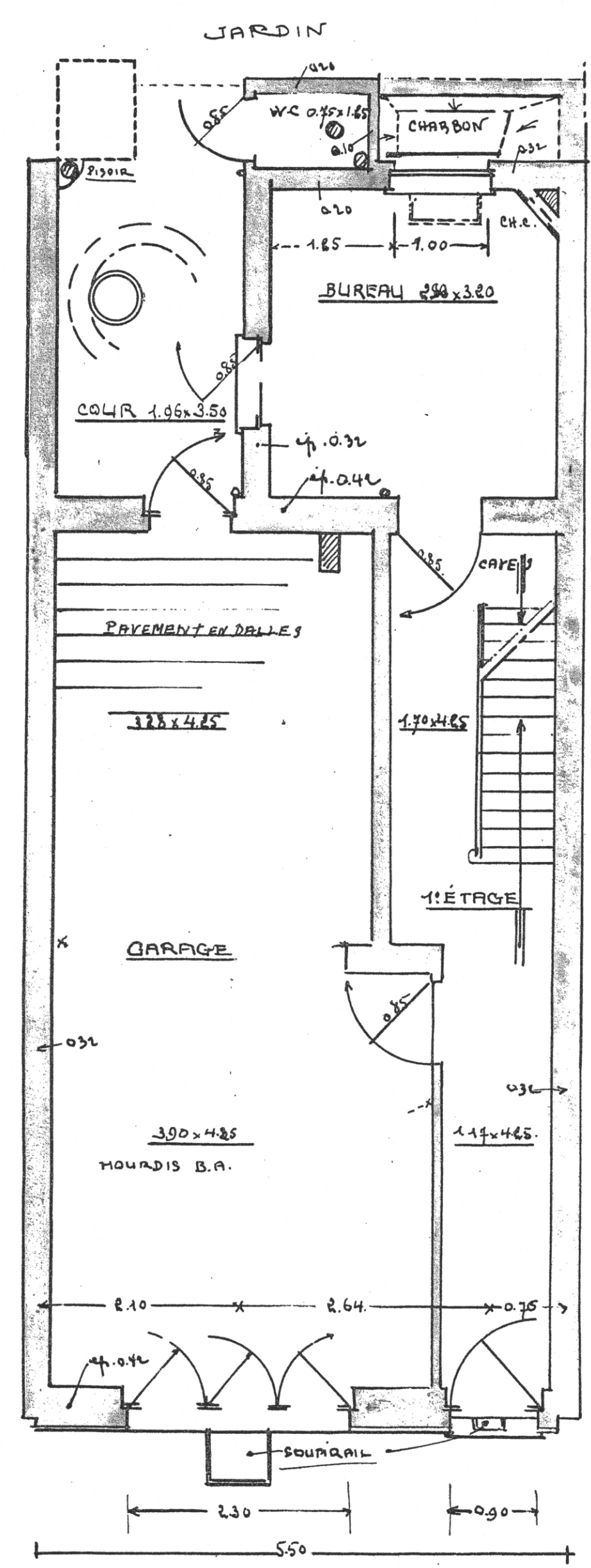
REZ-DE-CHAUSSEE
