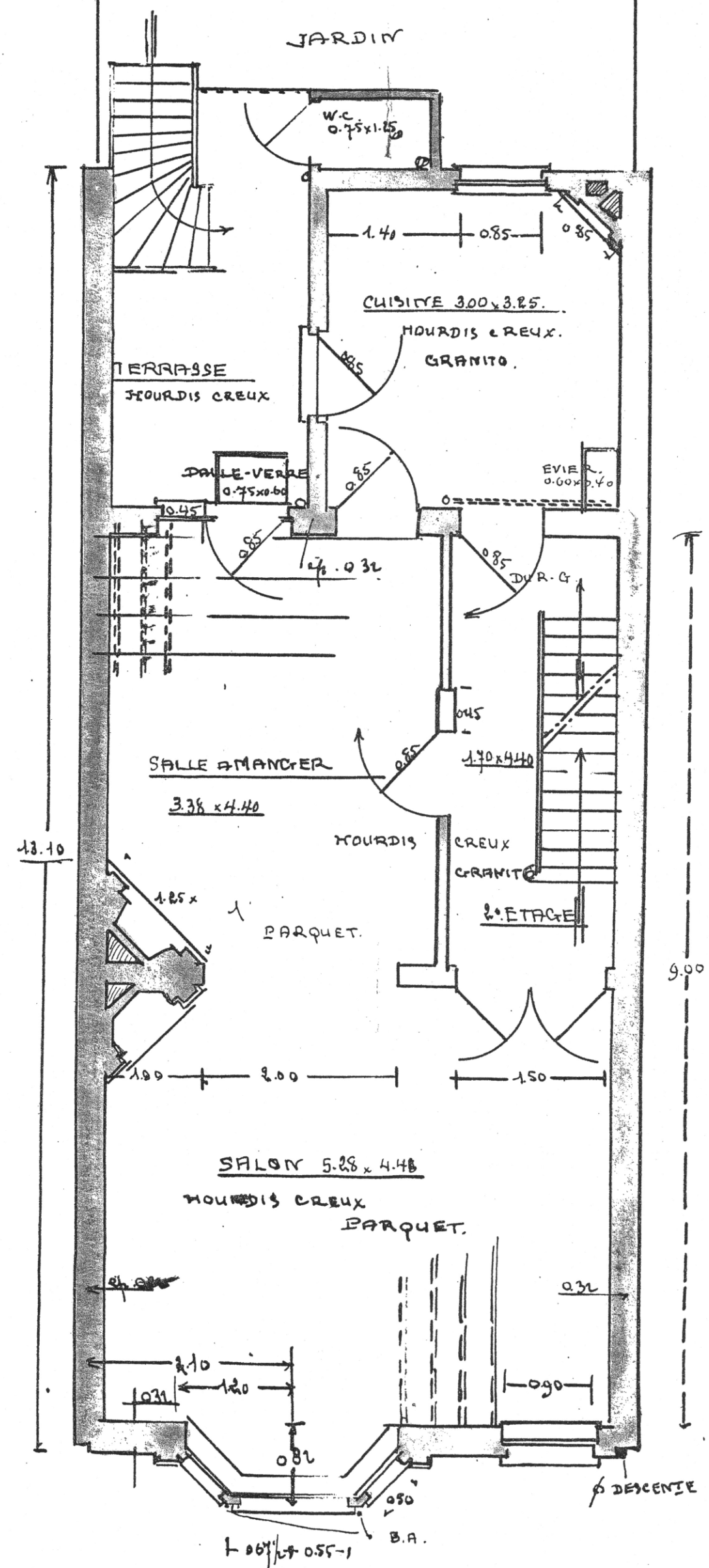
1 er ETAGE
