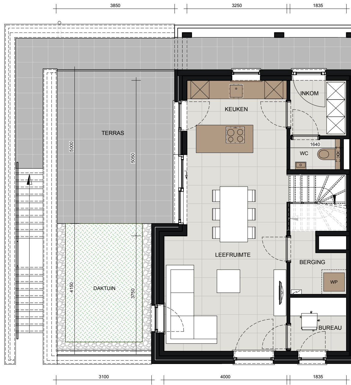
GRONDPLAN +01
