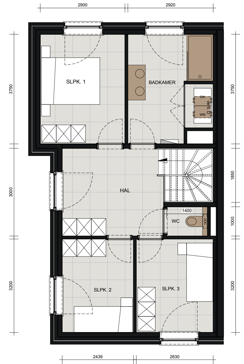
GRONDPLAN +02
