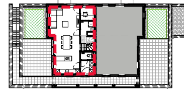
VERDIEPINGSPLAN +01
