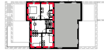
VERDIEPINGSPLAN +02
