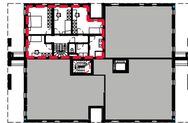
VERDIEPINGSPLAN +01
