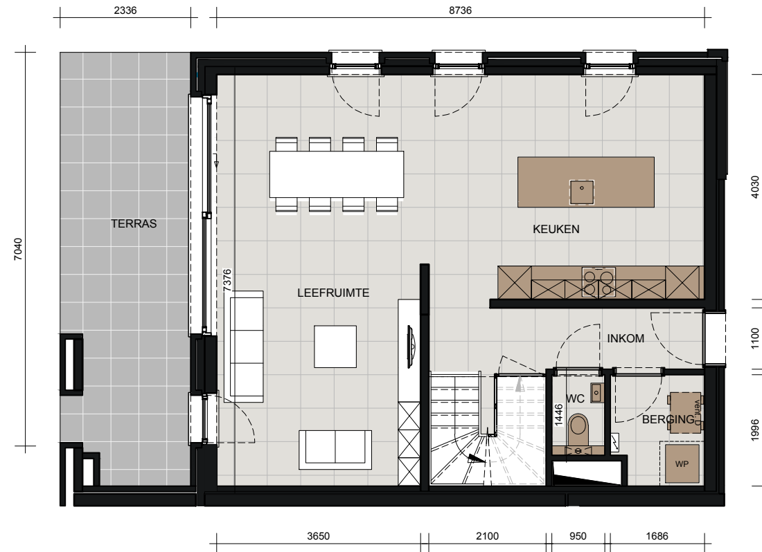
GRONDPLAN +00
