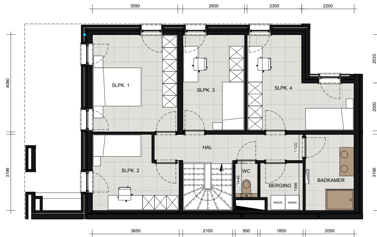
GRONDPLAN +01
