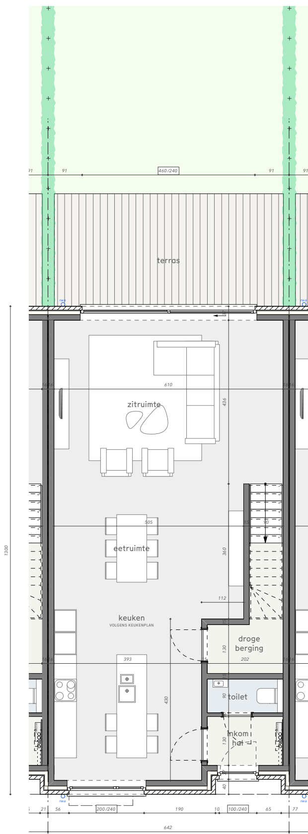
grondplan gelijkvloers
