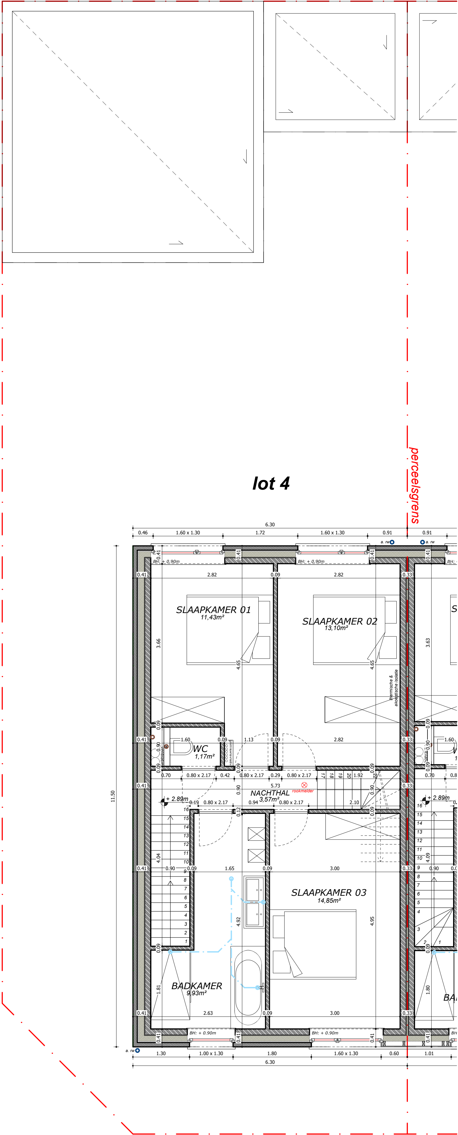
eerste verdieping schaal 1:50 lot 4 - 5 0 1 2 3 4 5
