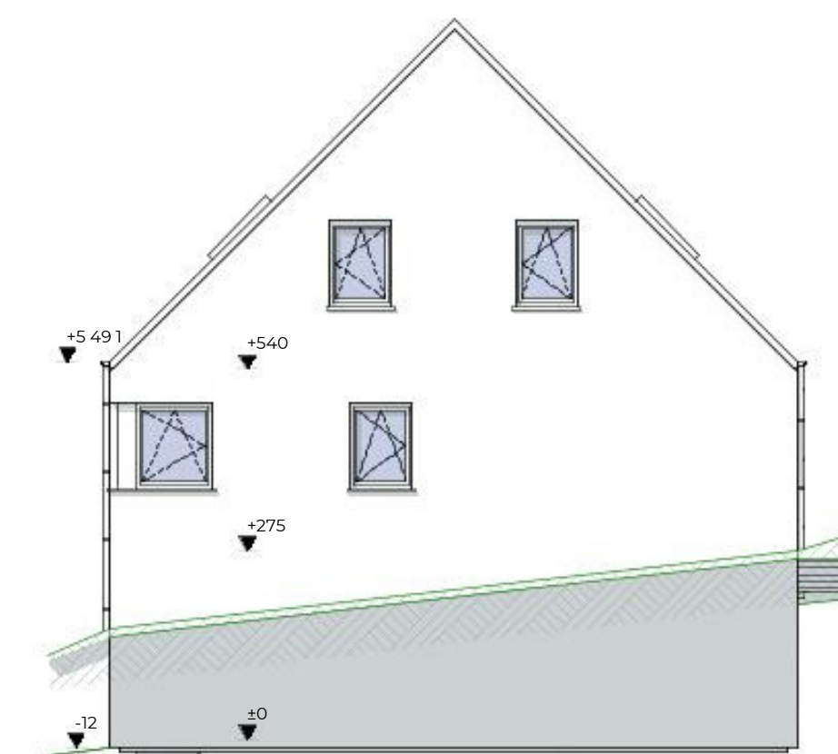
ZIJGEVEL RECHTS
