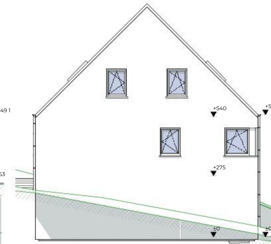
ZIJGEVEL LINKS
