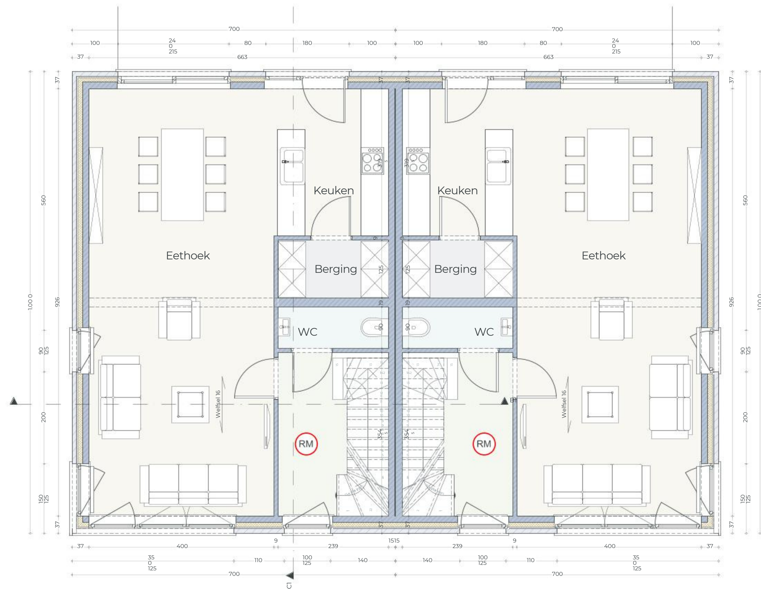
GELIJKVLOERS
