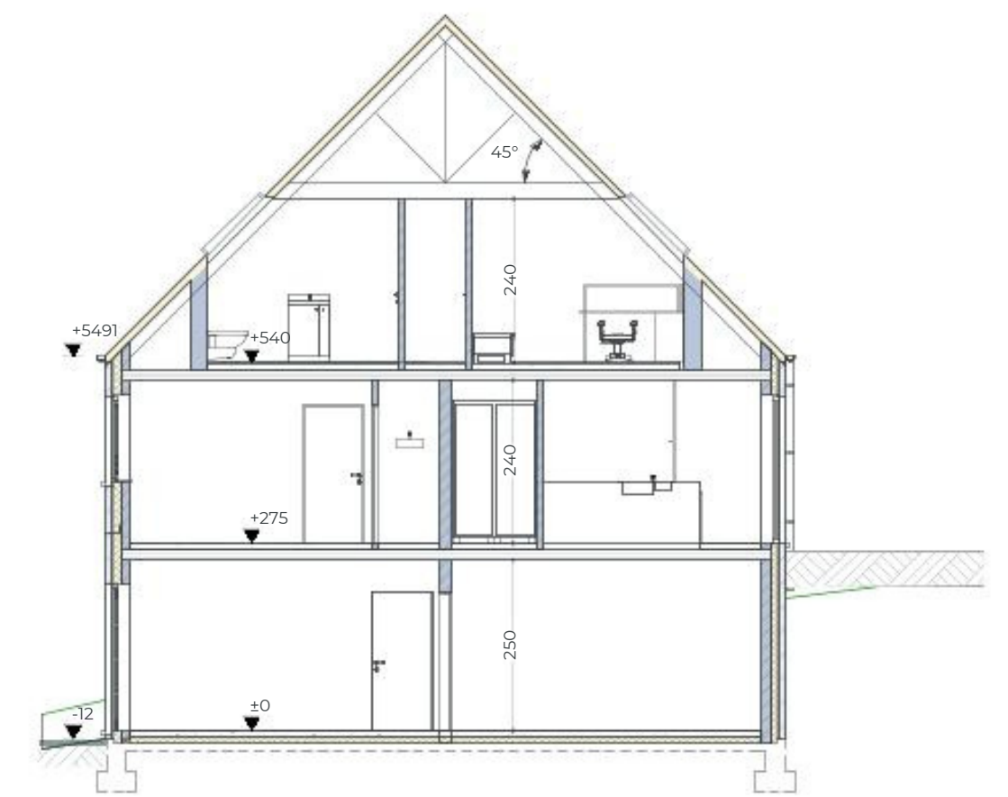
DOORSNEDE
