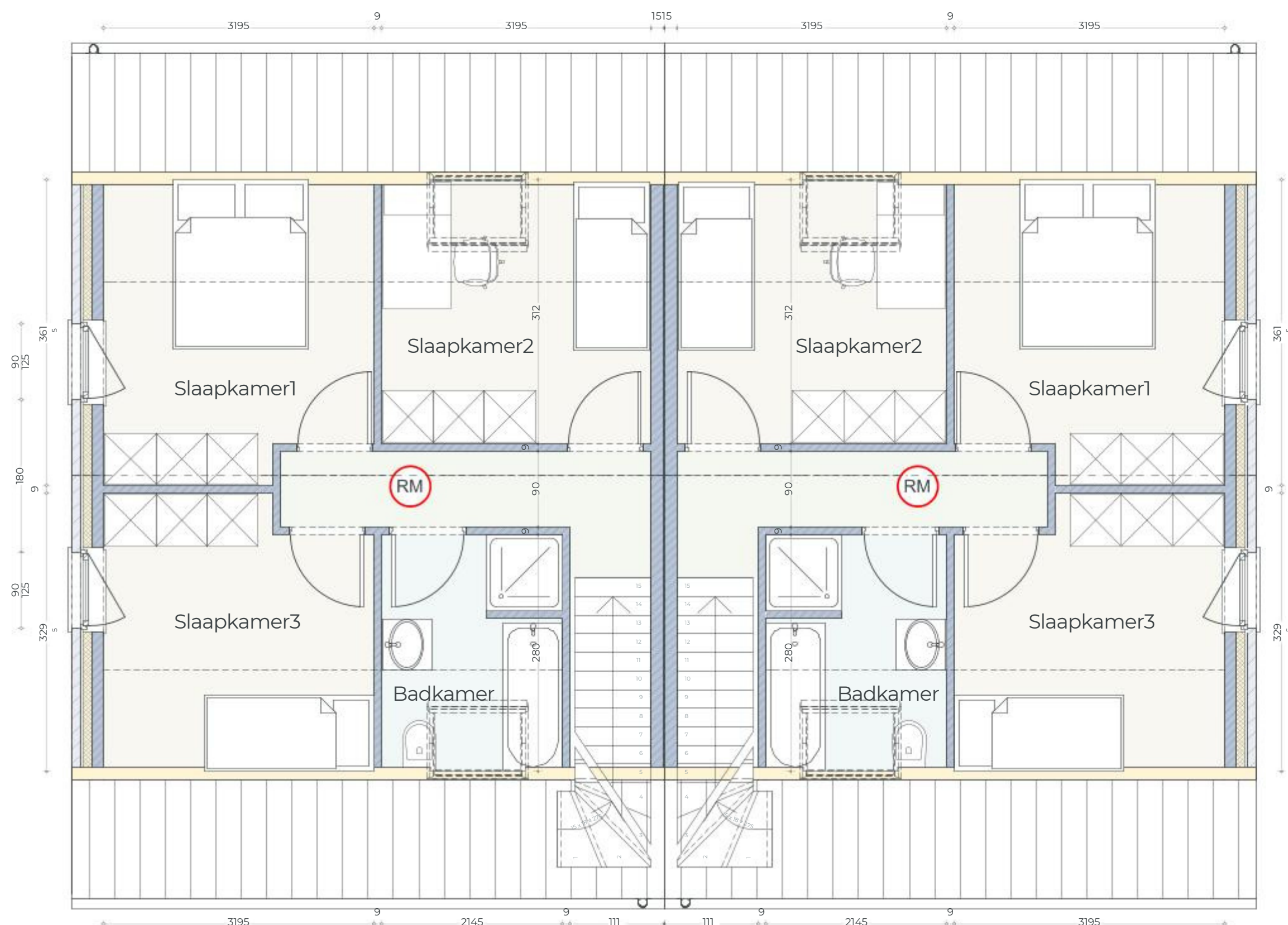
VERDIEPING
