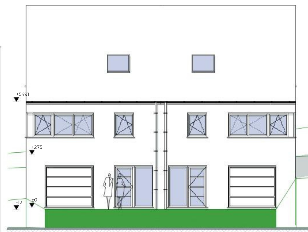
VOORGEVEL
