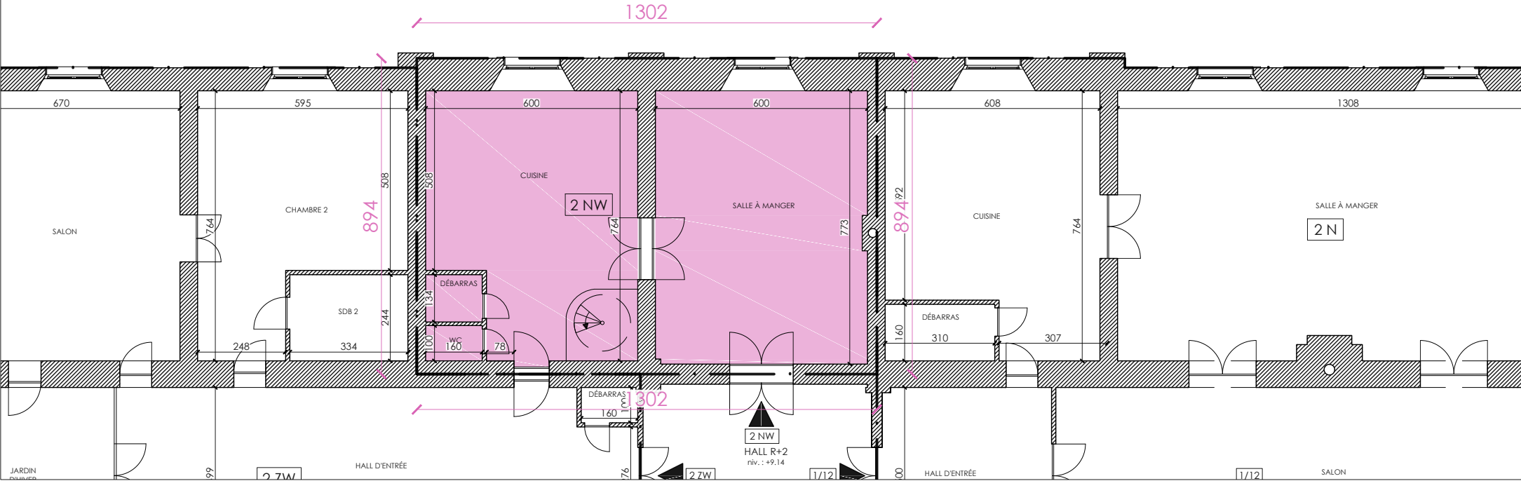
R+2 PLAN DU LOGEMENT 1/150 N
