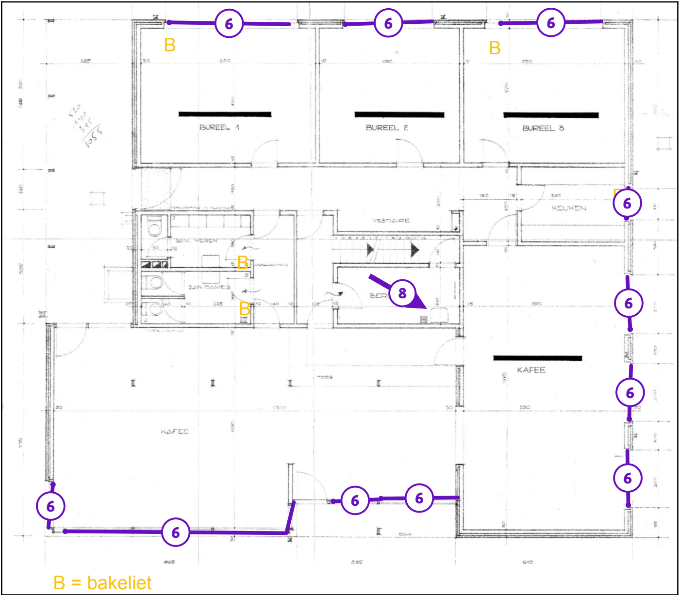
Legende van plan 1.4: café
