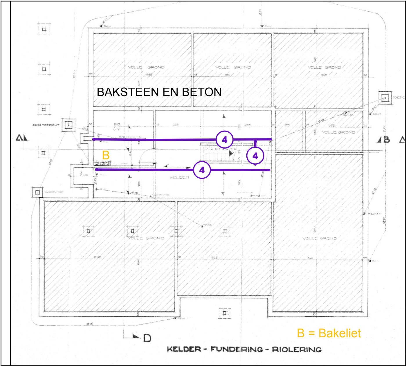
Legende van plan 1.1: kelder - café
