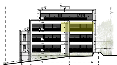
ACHTERGEVEL
