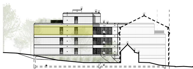
LINKERZIJGEVEL
