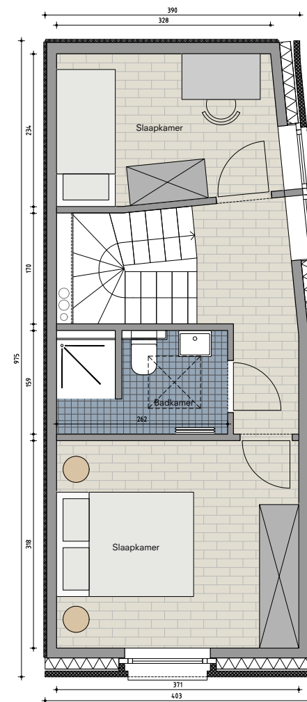
TWEDE VERDIEPING
