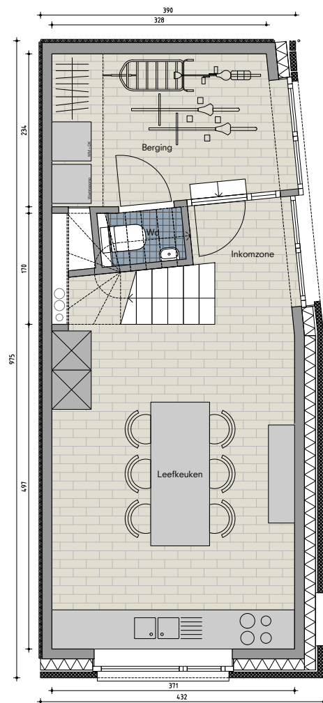
GELUKVLOERSE VERDIEPING
