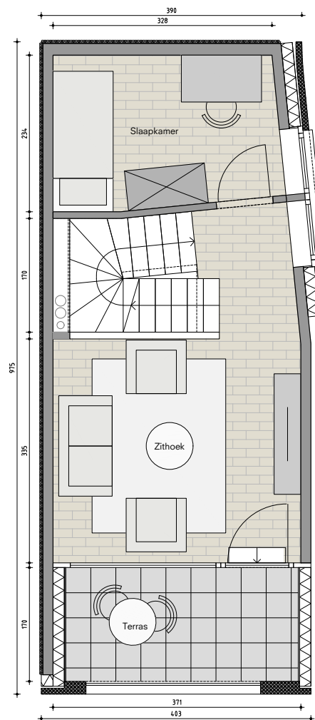
EERSTE VERDIEPING
