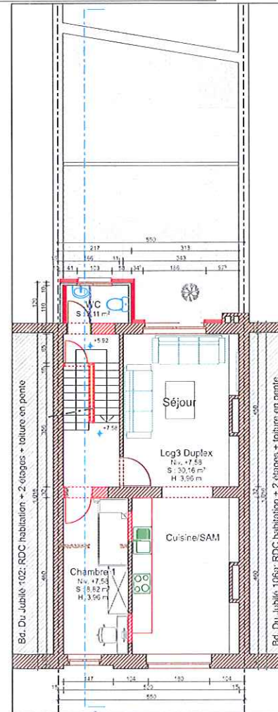
2. 2ème ETAGE 1:50
