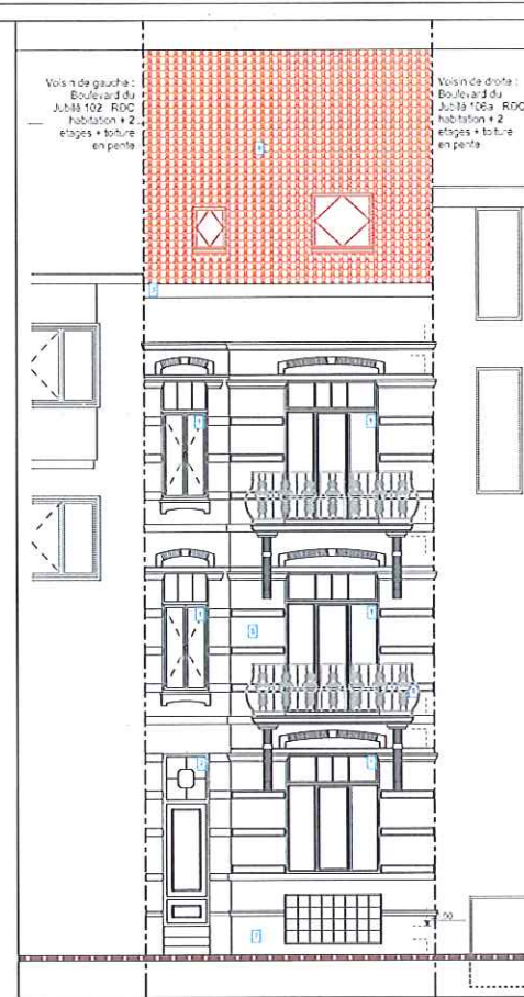
FACADE AVANT 1:50
