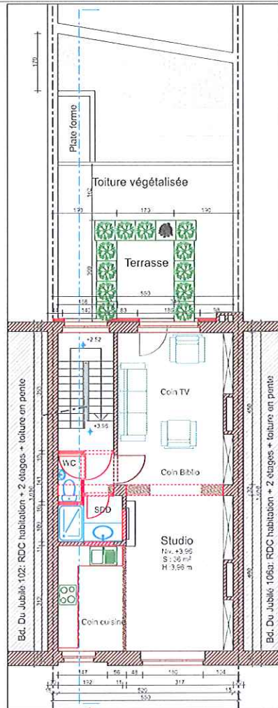
1. 1er ETAGE 1:50
