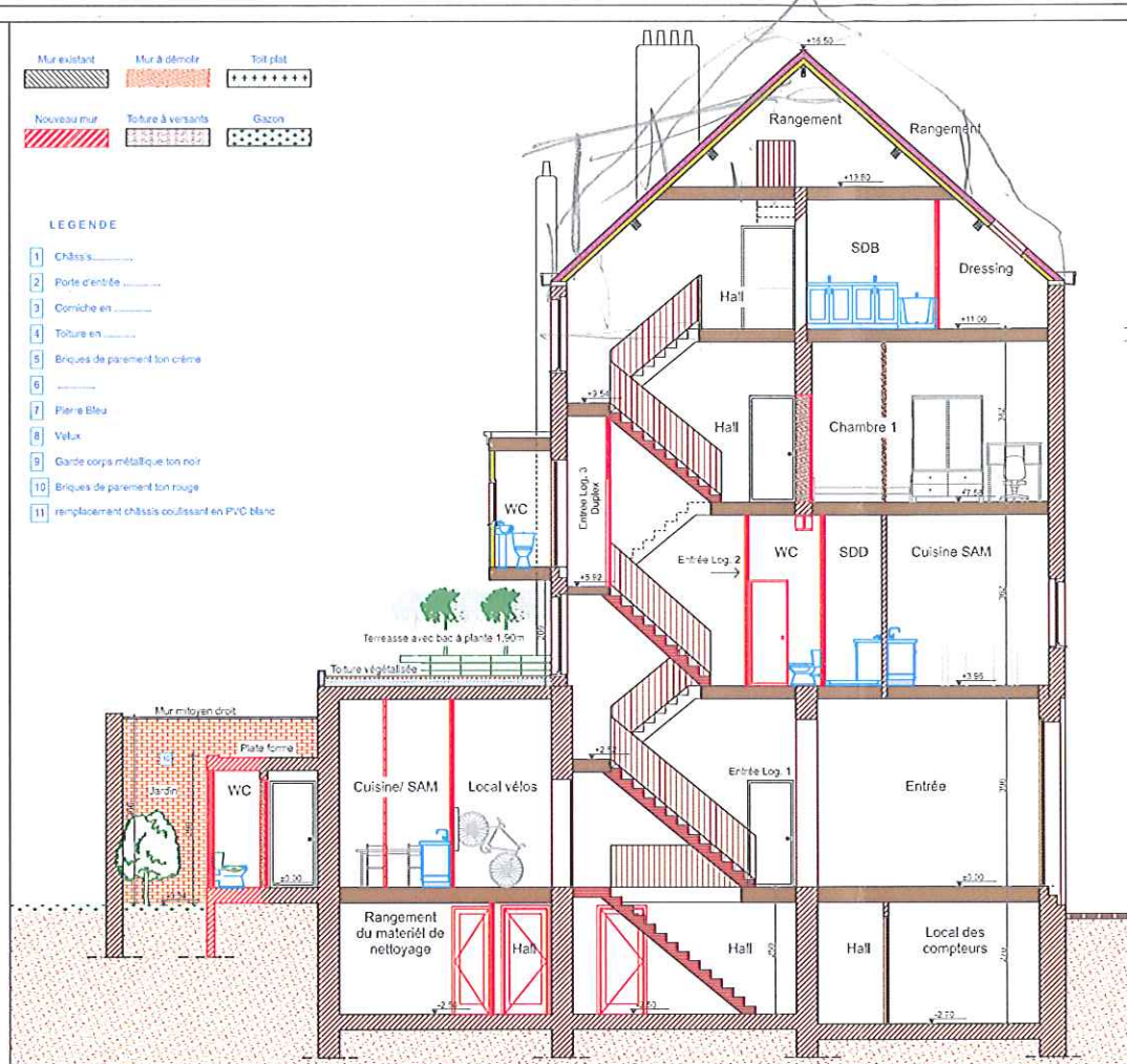
COUPE AA 1:50
