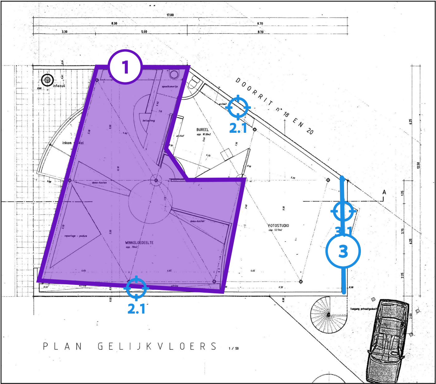
Legende van plan 1.1: Handelsgelijkvloers plan
