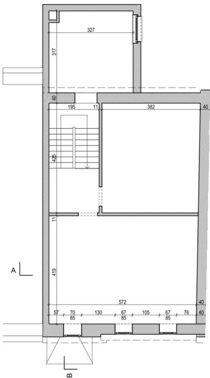
Situation existante - plan du 2ème étage
