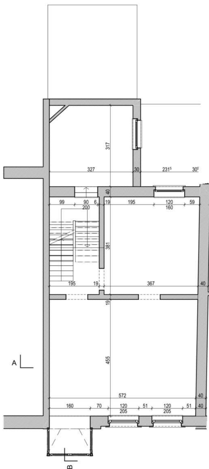
Situation existante - plan du 1er étage
