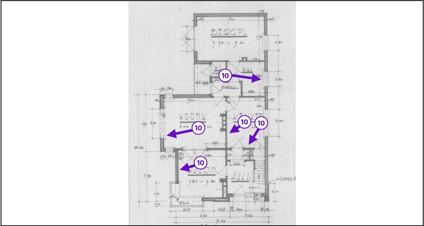
Legende van plan 2.10: gelijkvloers
