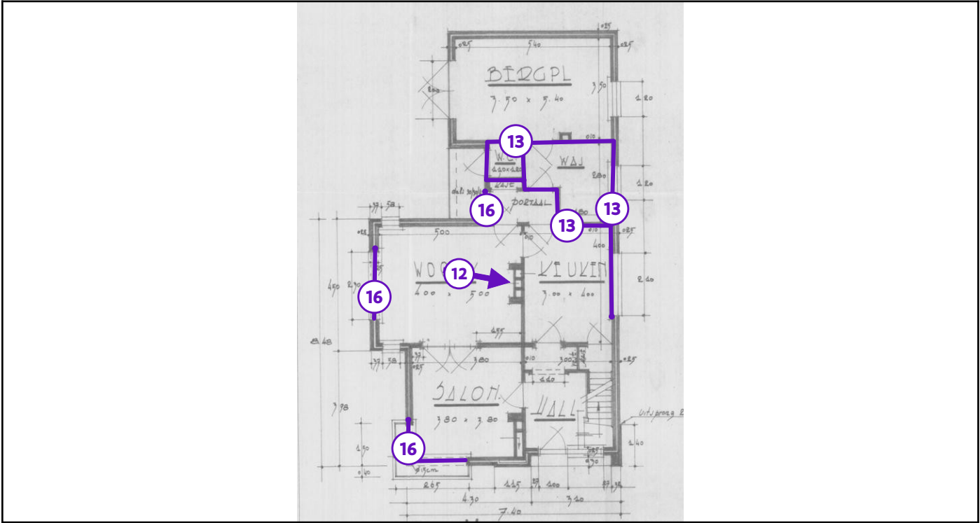
Legende van plan 2.8: gelijkvloers
