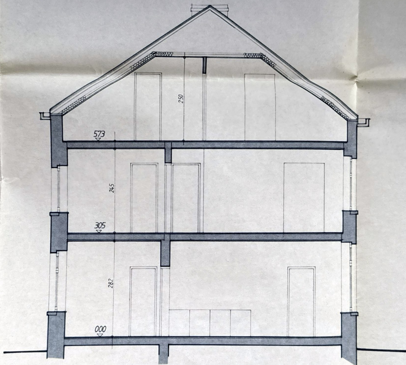
COUPE A.A
