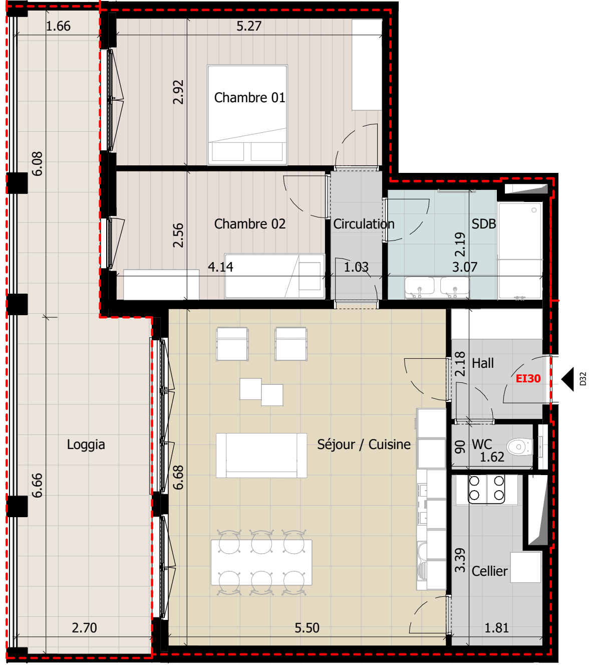
Plan de vente_Appartement D32 Ech: 1 : 75
