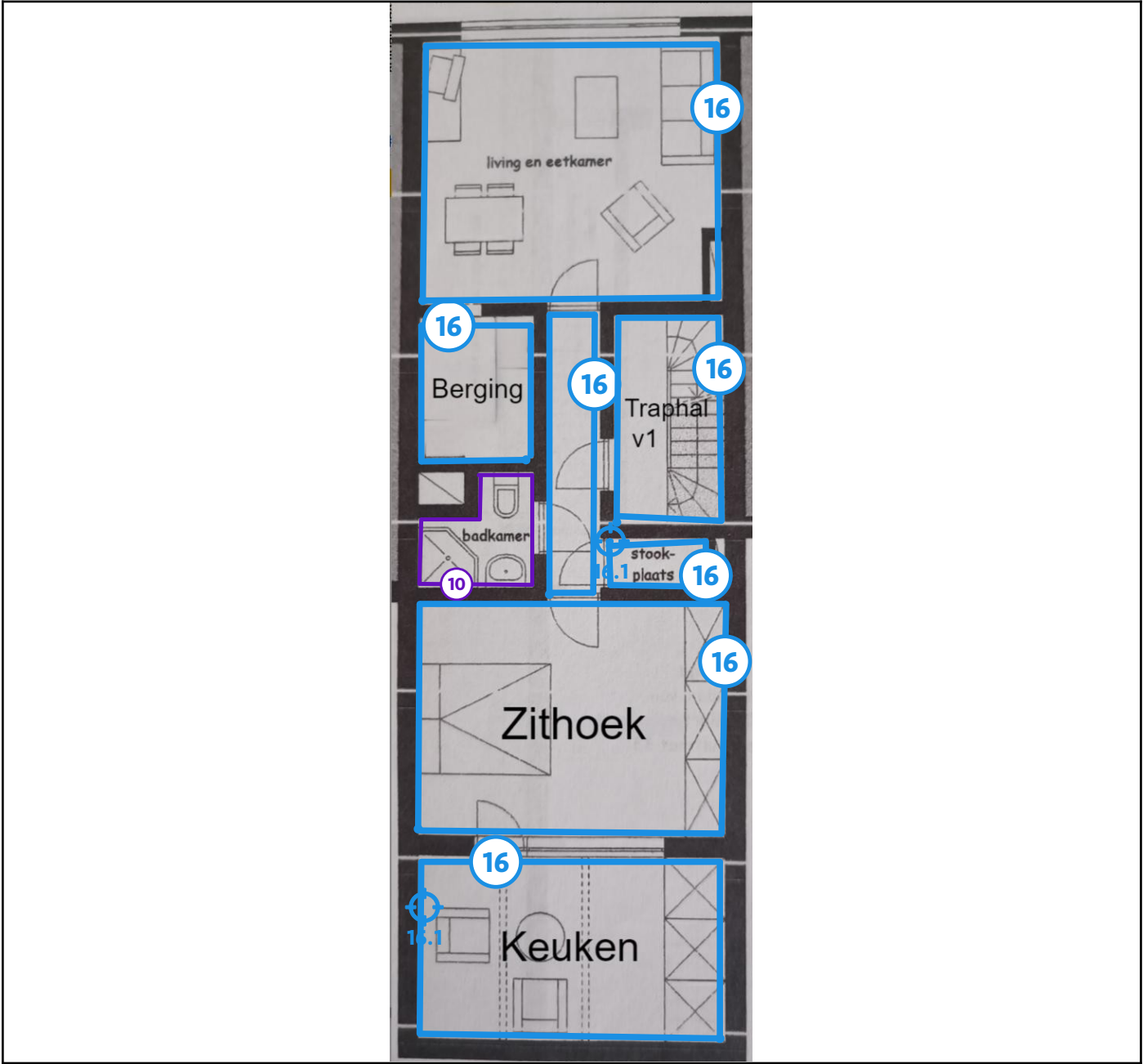
Legende van plan 1.7: Verdiep 1 - aanduiding muren
