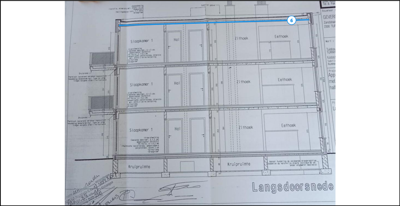
Legende van plan 1.2: Doorsnede plan
