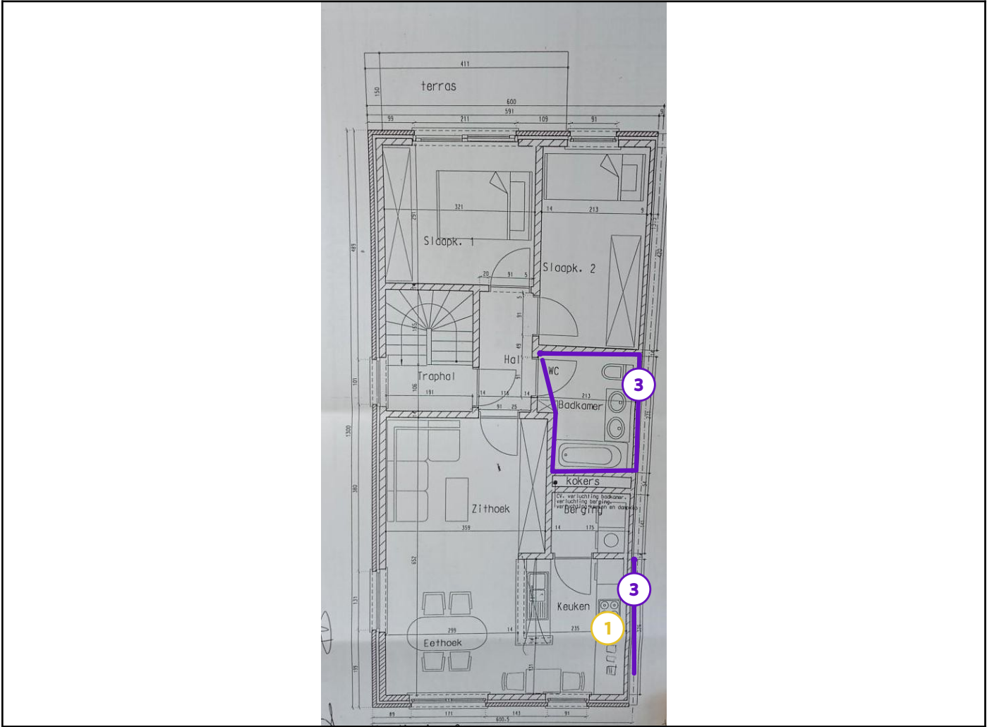
Legende van plan 1.3: Grondplan appartement
