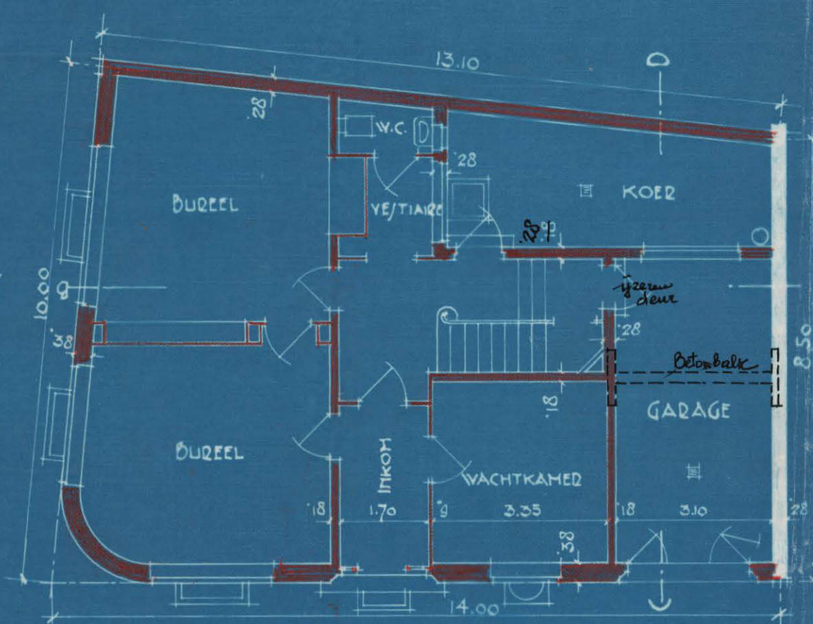
GEELIJKVLOER/
