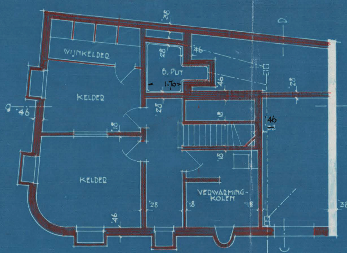
KELDERING
