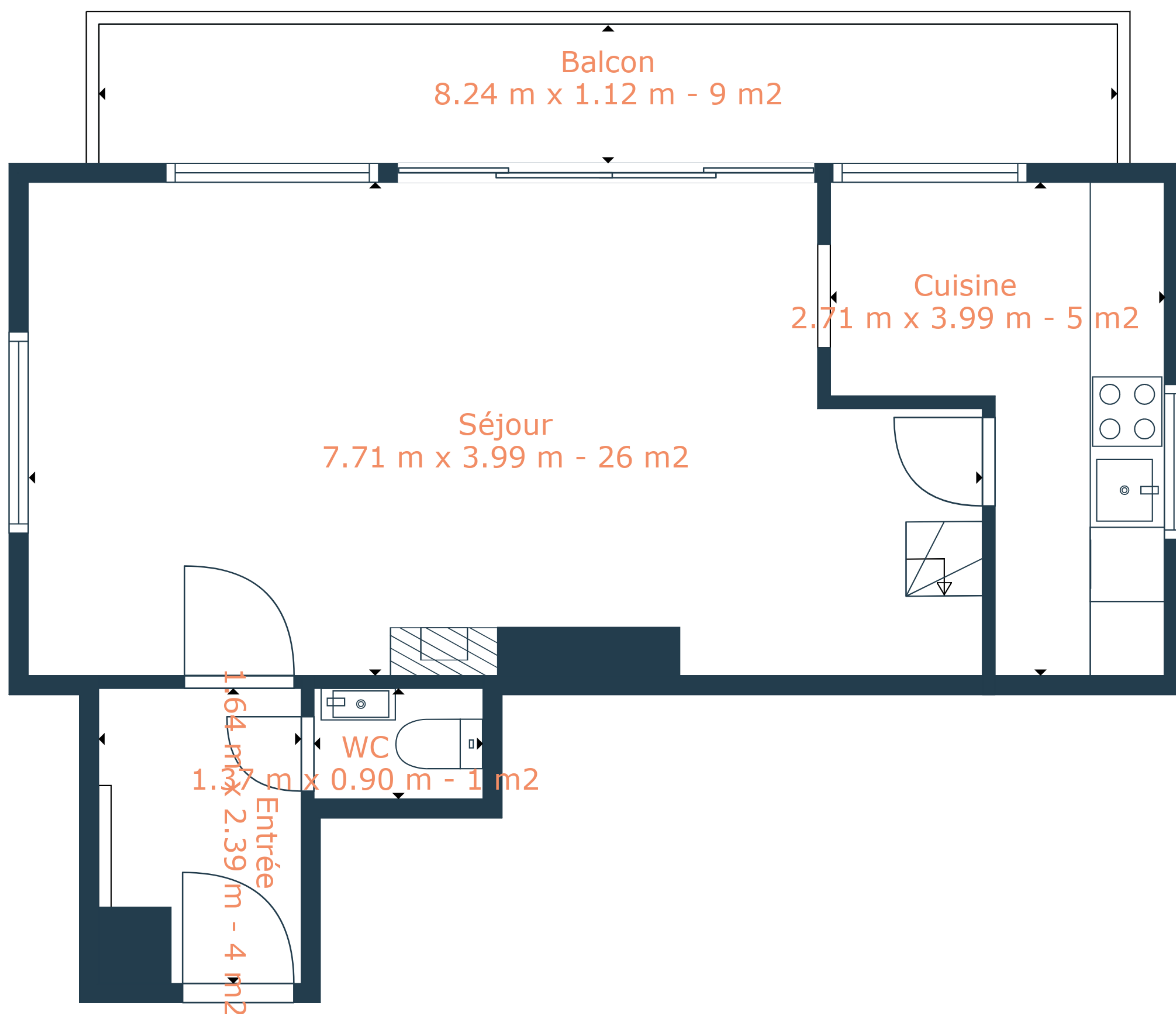
1er Étage
