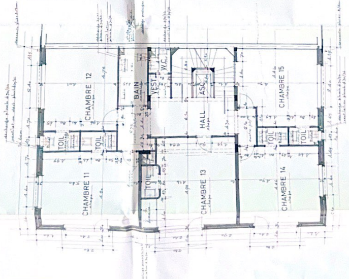
2eme ETAGE
