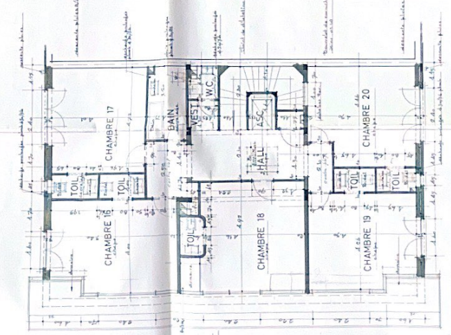
3eme ETAGE
