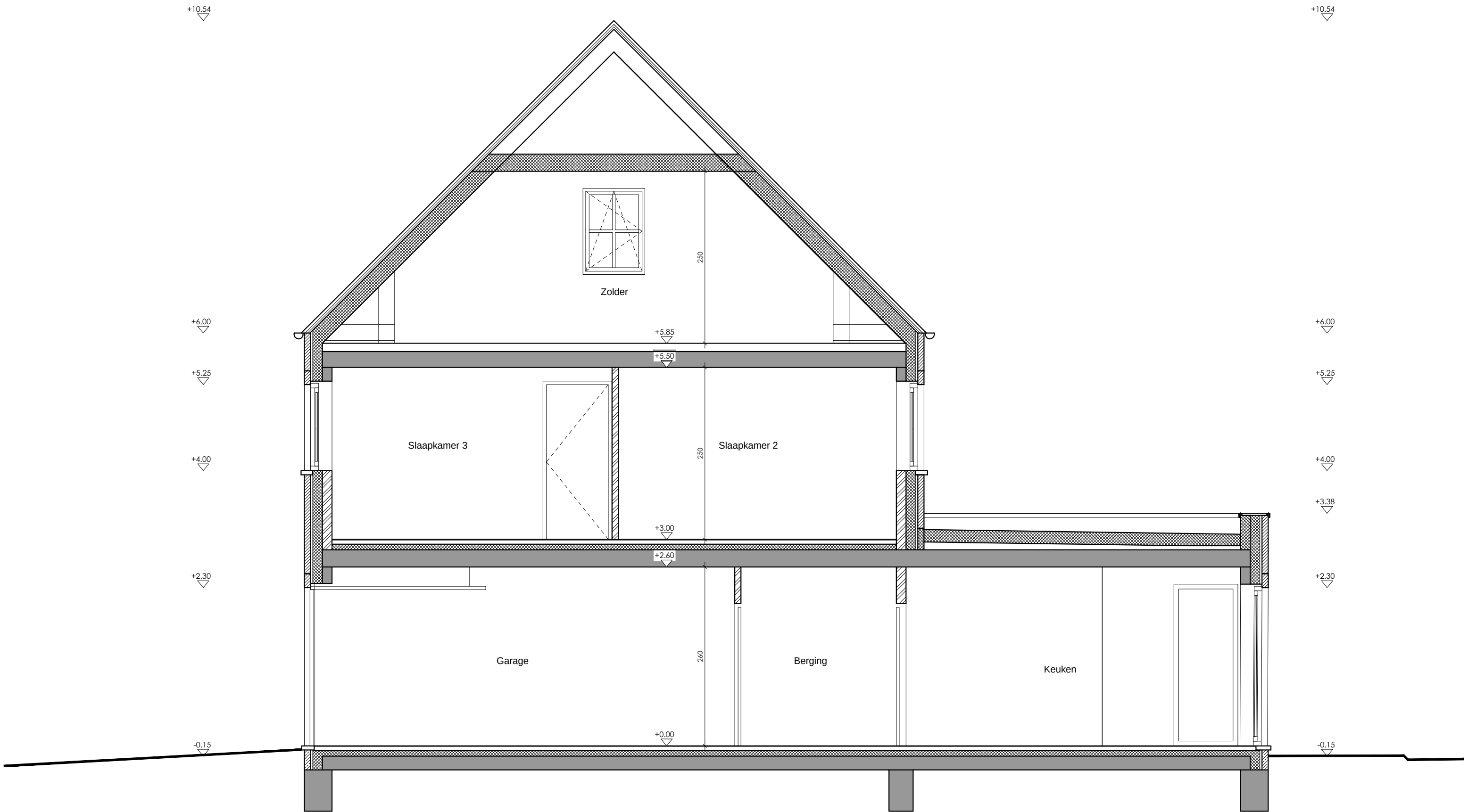
Snede A-A BOSSTRAAT Lot 1 tem 4
