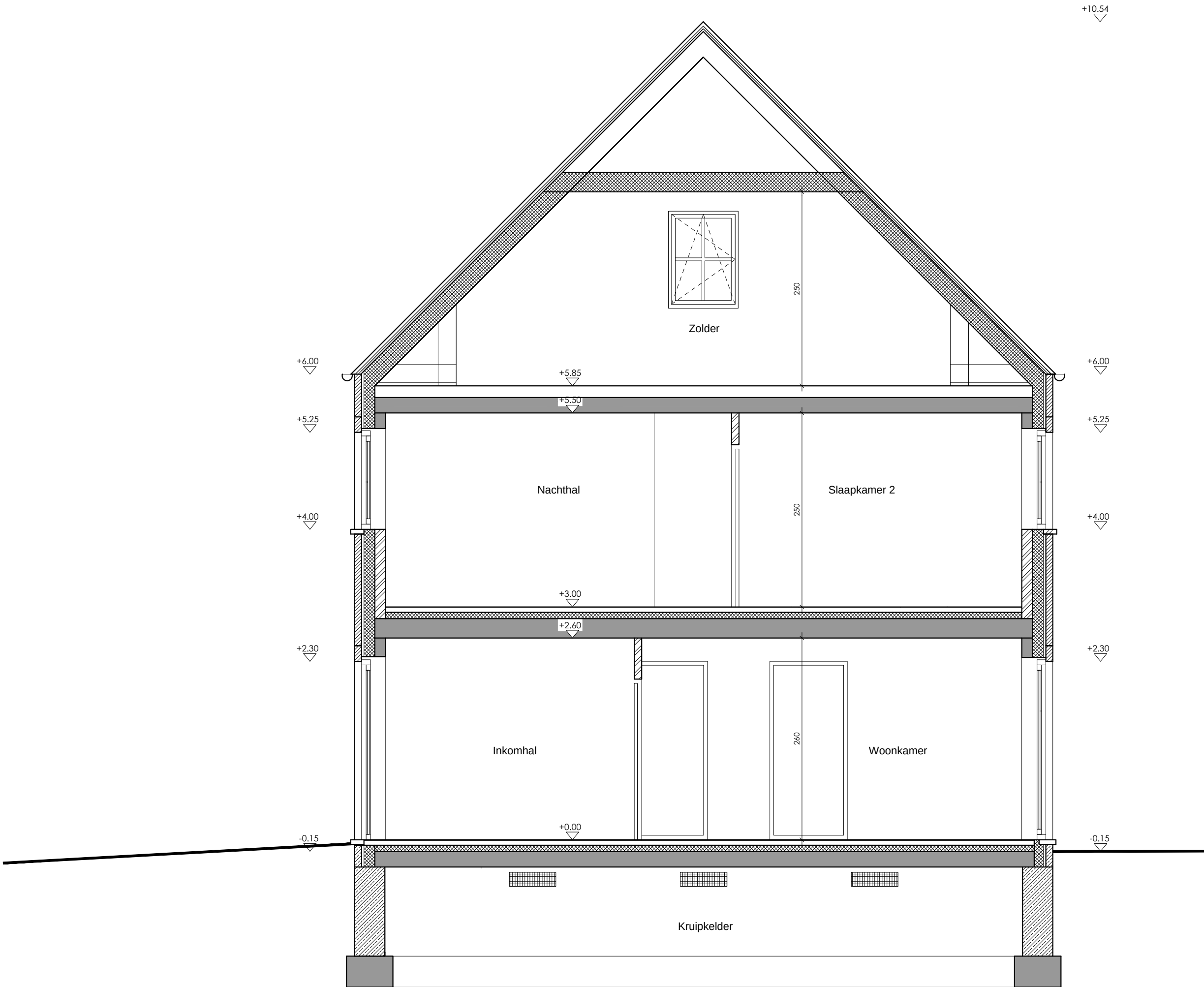
Snede B-B
