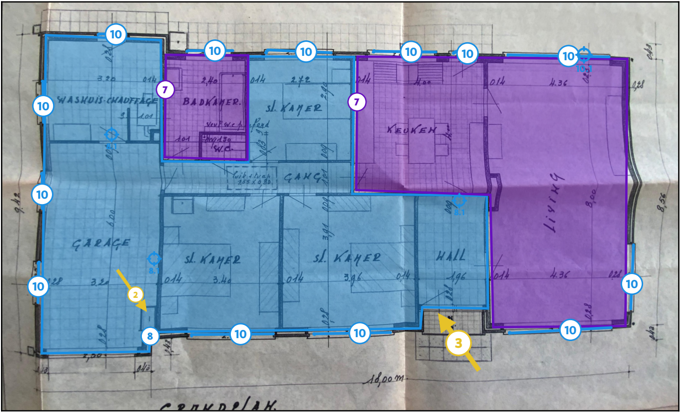
Legende van plan 1.2: Grondplan glv
