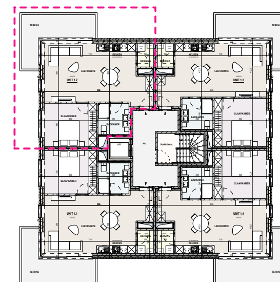
VERDIEPING 1
