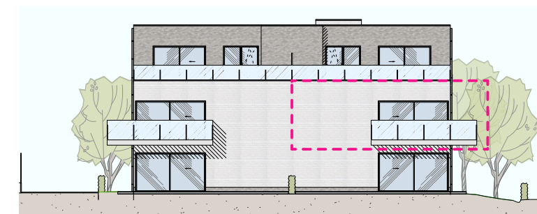
ACHTERGEVEL
