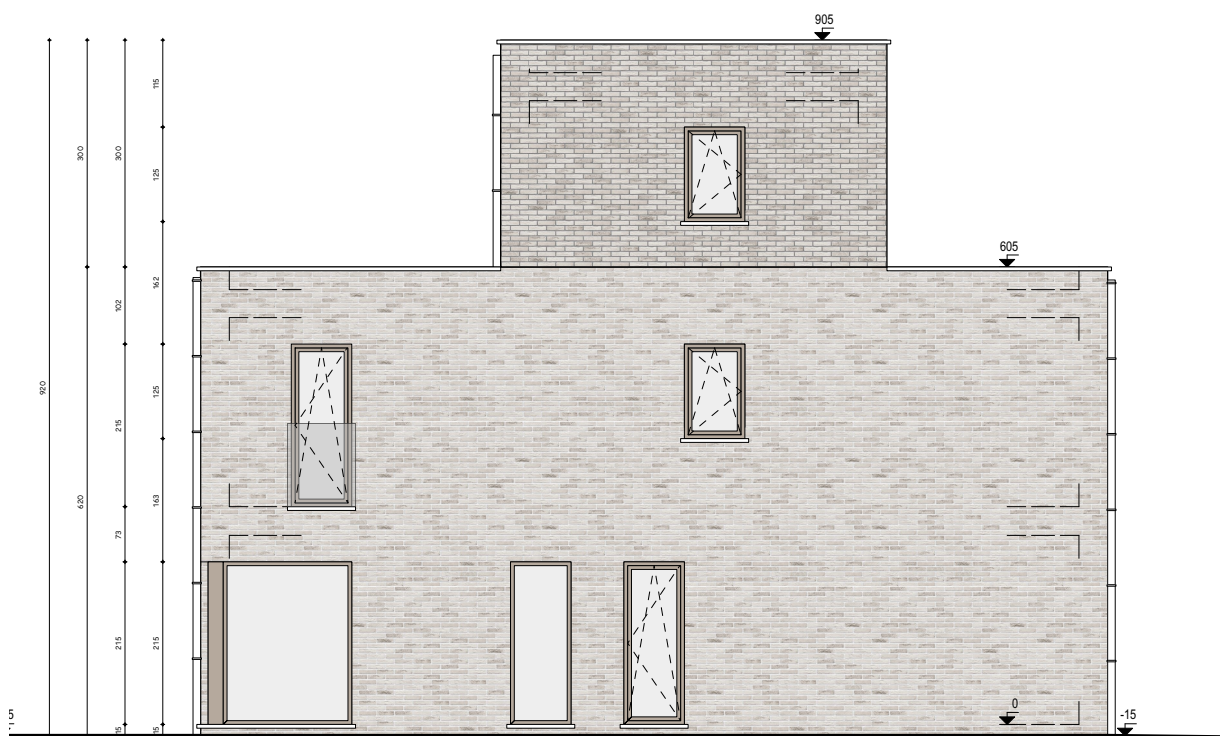
aanzicht linkergevel
