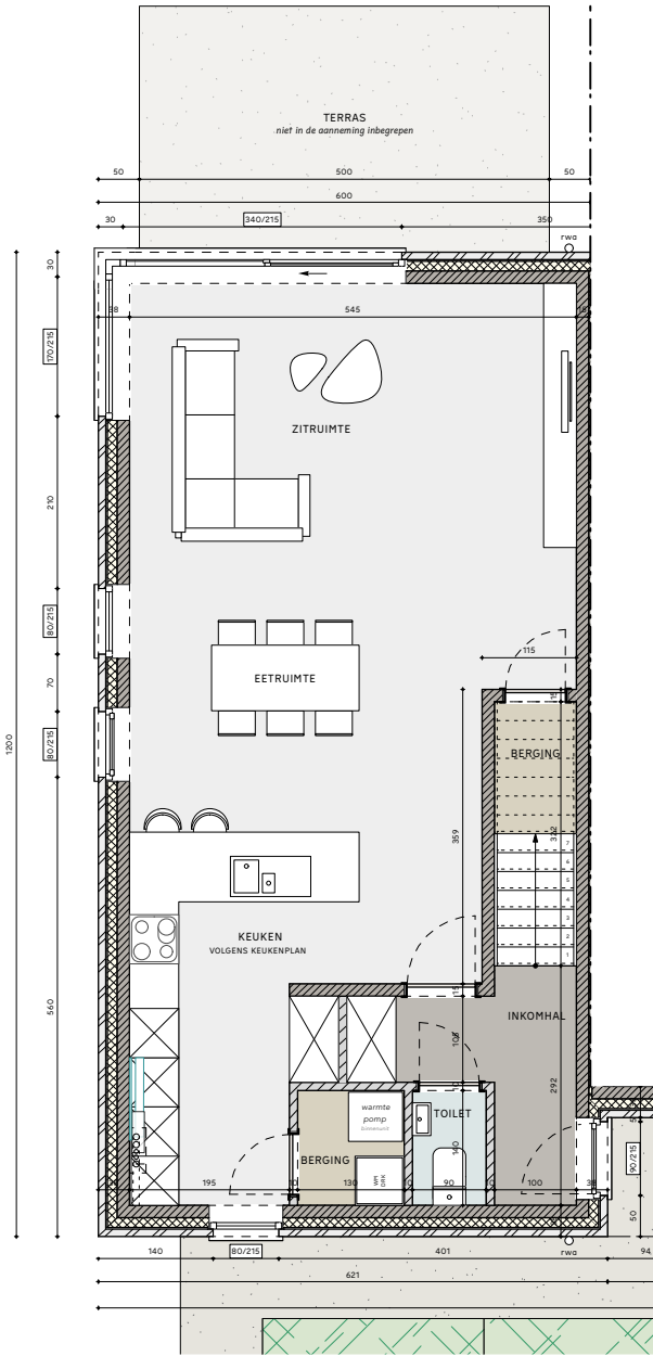
grondplan gelijkvloers
