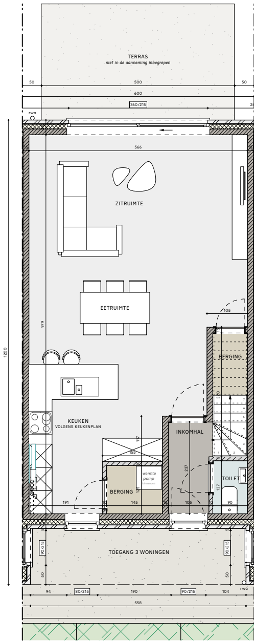
grondplan gelijkvloers
