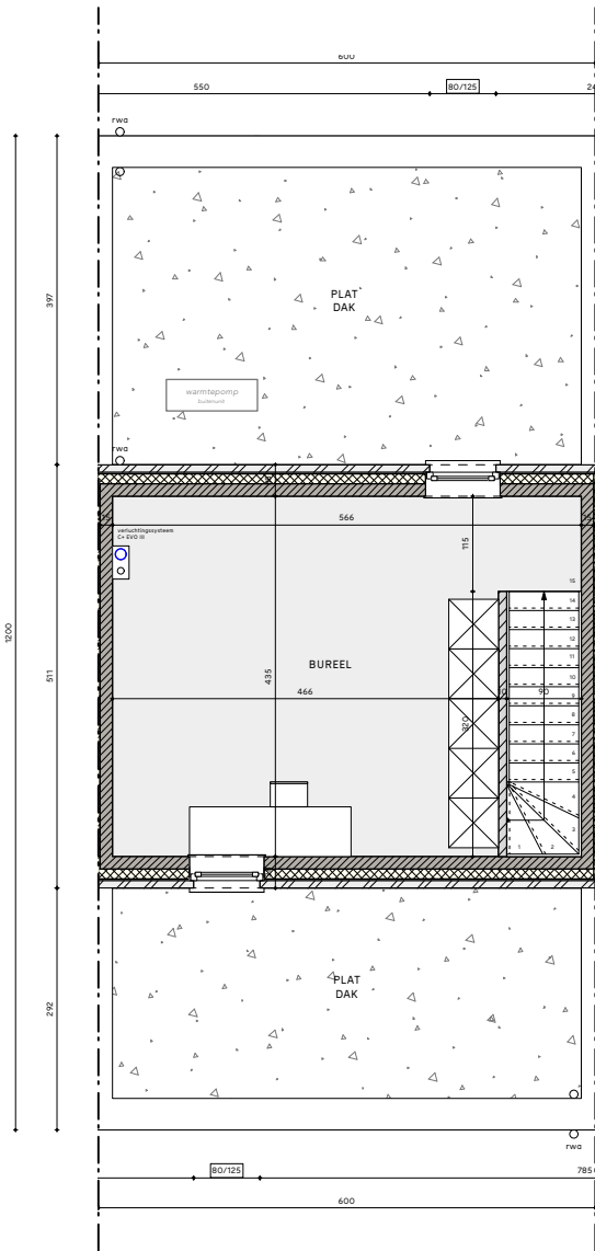
grondplan zolder
