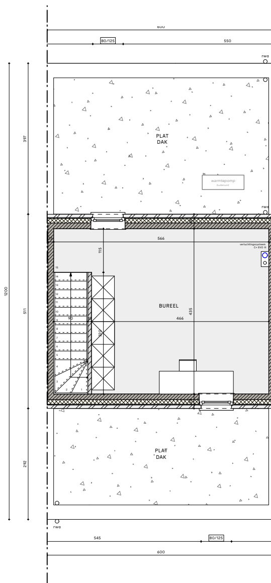
grondplan zolder
