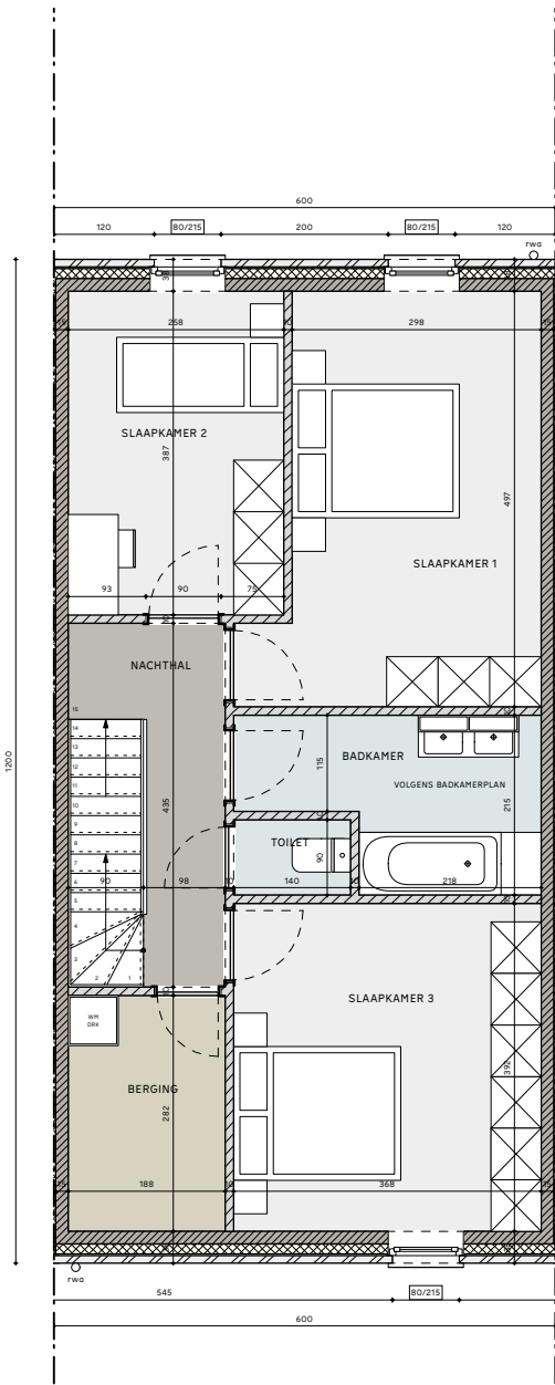
grondplan verdieping
