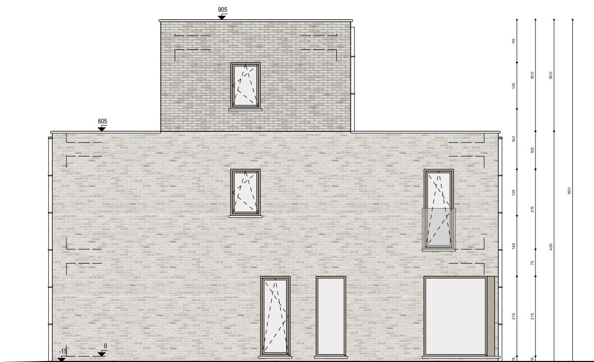
aanzicht rechtergevel
