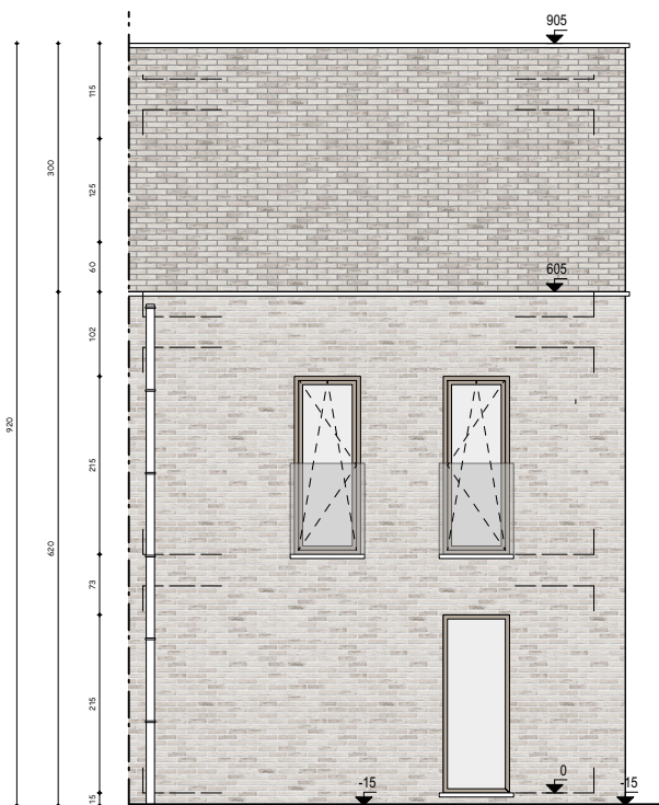
aanzicht voorgevel
