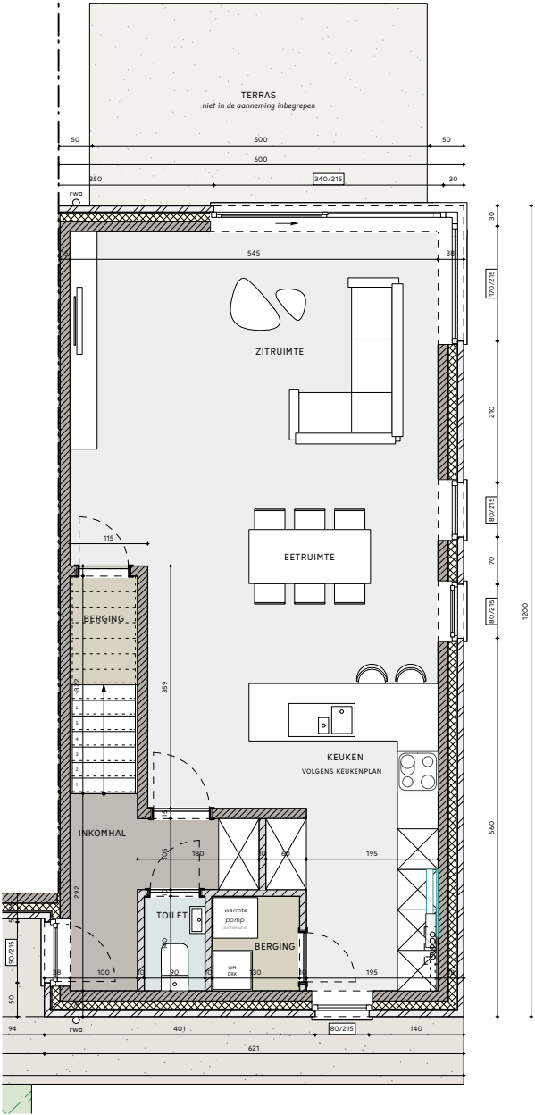
grondplan gelijkvloers
