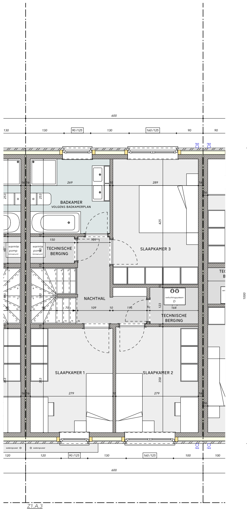
GRONDPLAN verdieping
