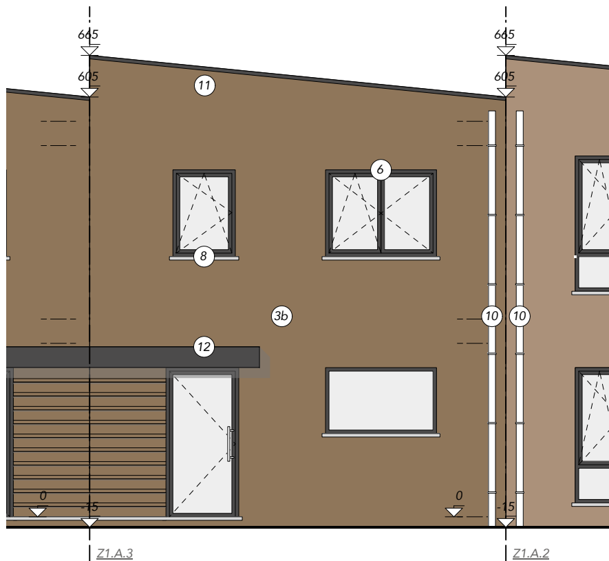
AANZICHT voorgevel
