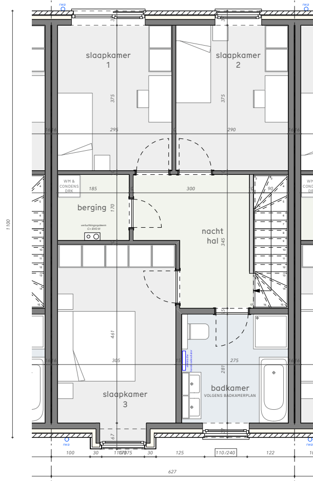
grondplan verdieping
