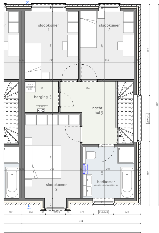
grondplan verdieping
