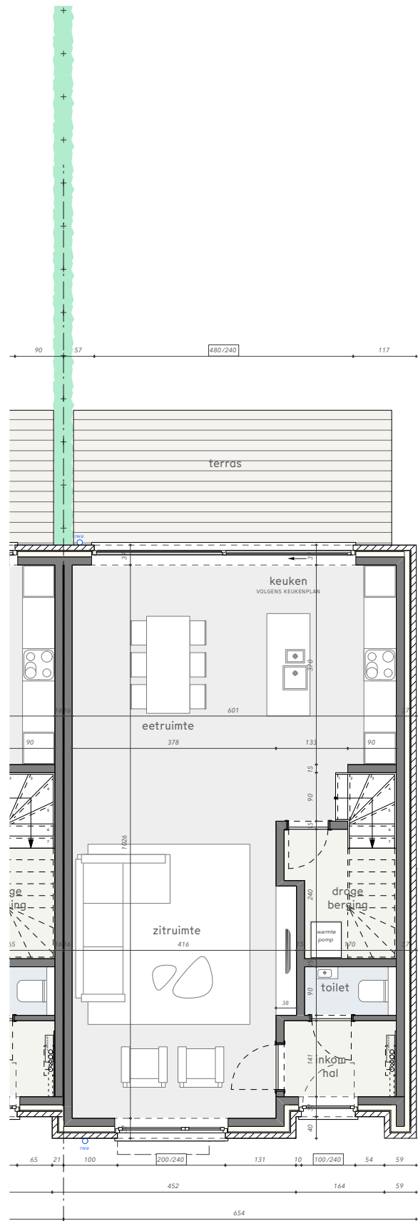
grondplan gelijkvloers
