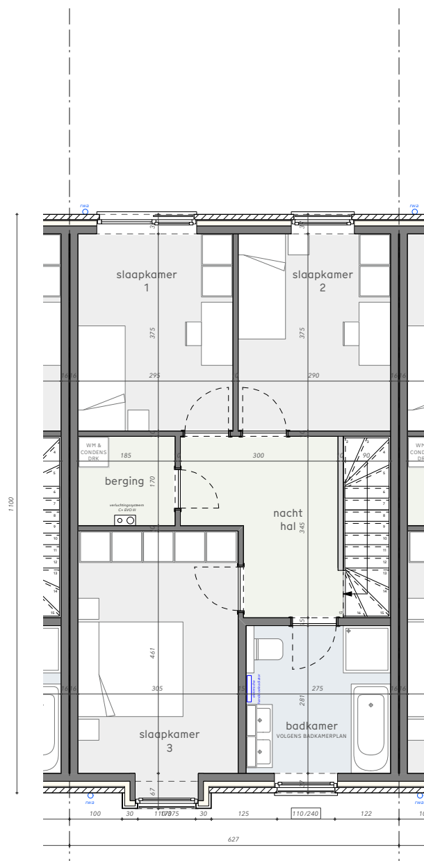
grondplan verdieping
