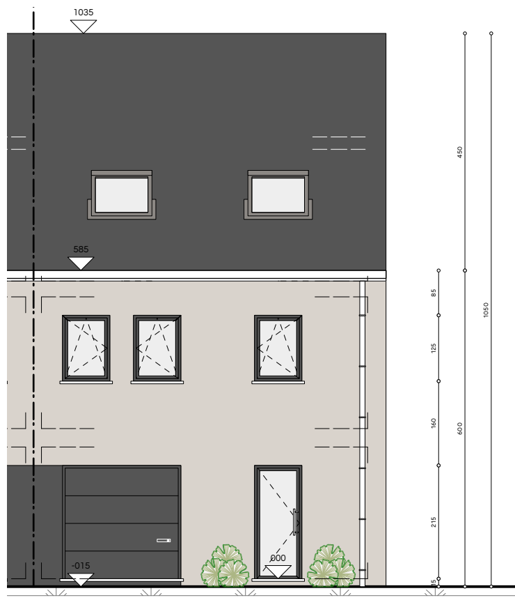
aanzicht voorgevel
