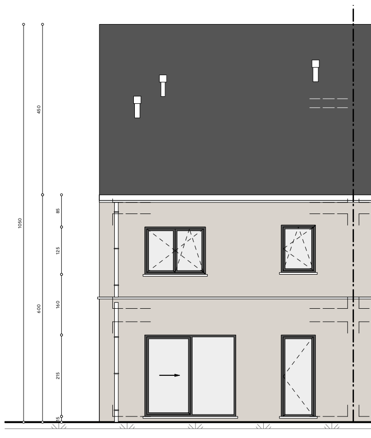
aanzicht voorgevel
