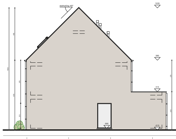
aanzicht zijgevel
