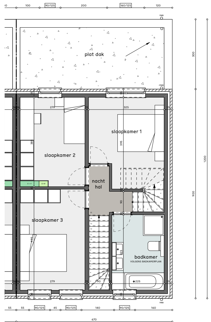
grondplan verdieping
