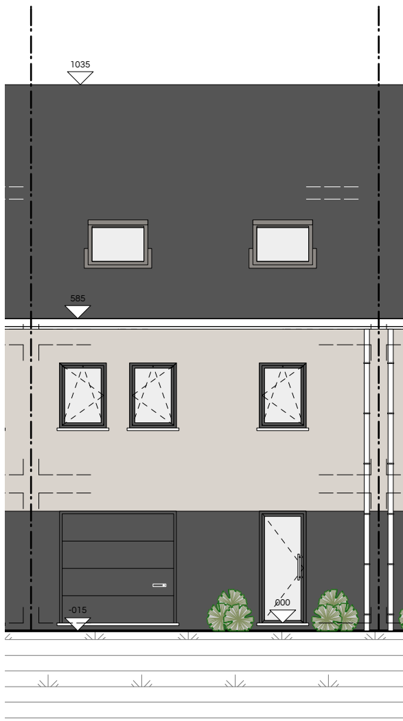
aanzicht voorgevel
