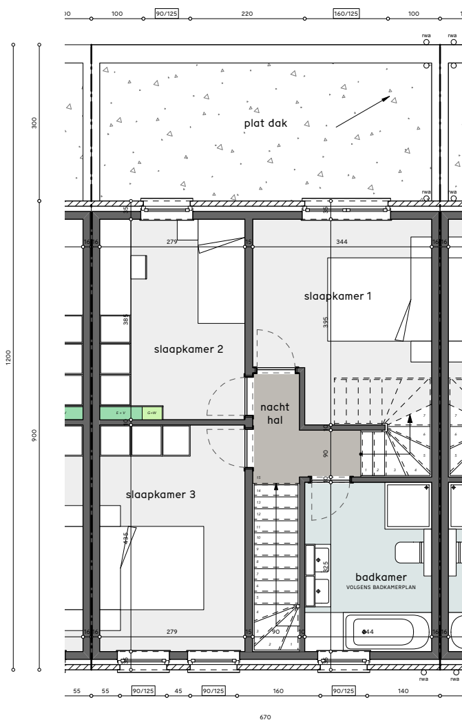
grondplan verdieping
