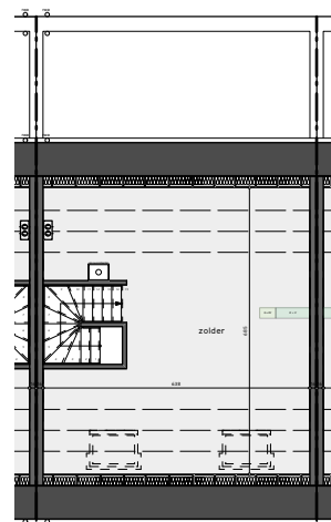
grondplan zolder
