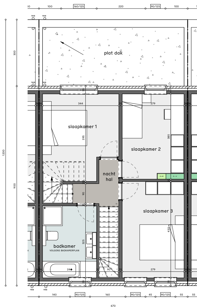
grondplan verdieping
