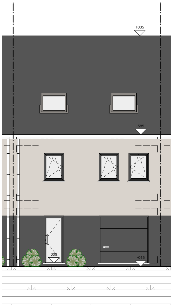
aanzicht voorgevel
