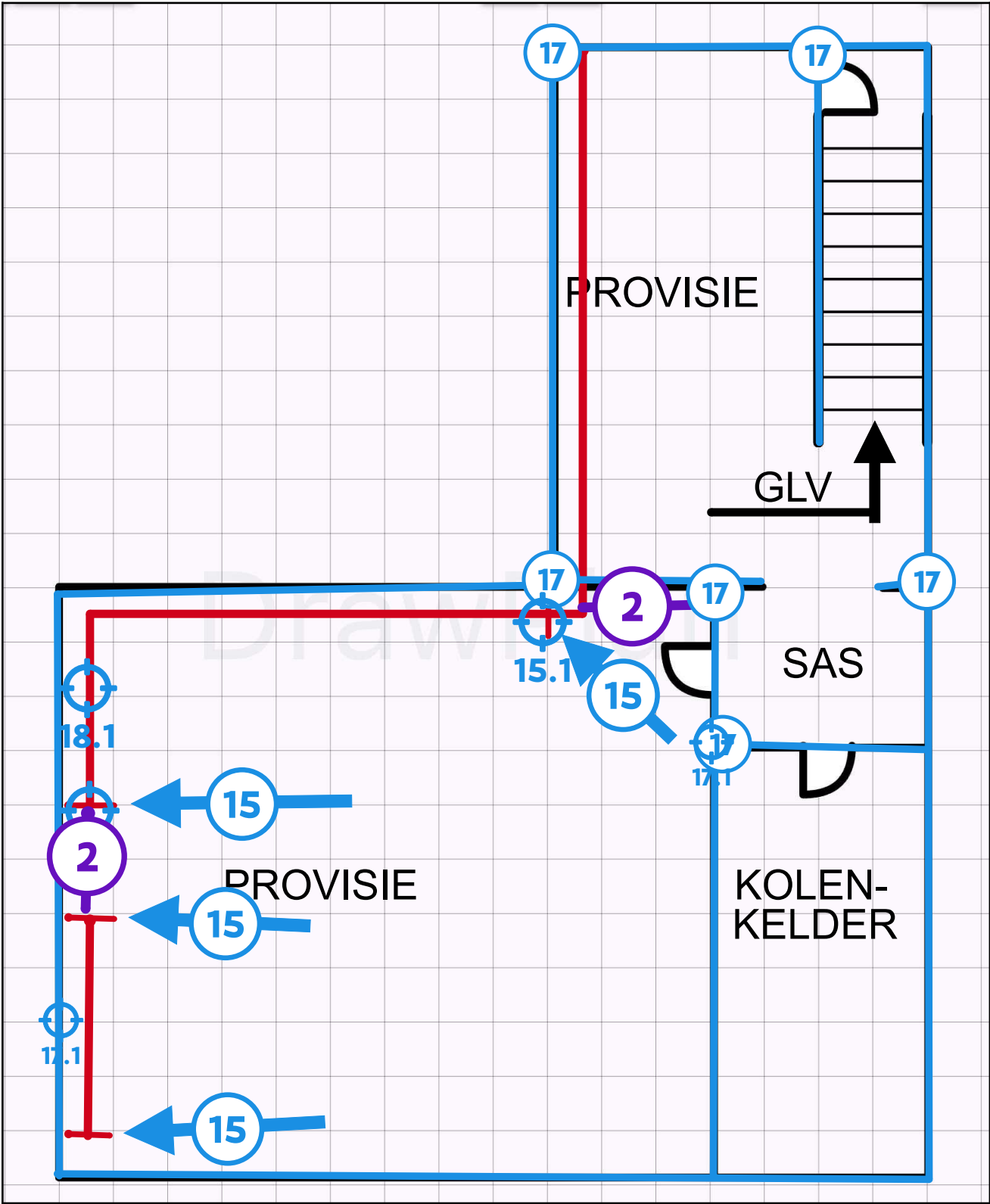
Legende van plan 1.4: KELDER
