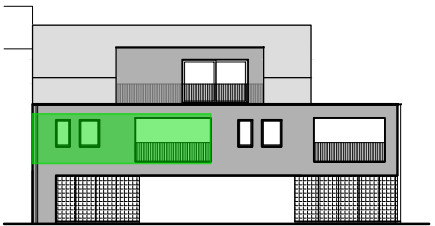
ACHTERGEVEL - Z
