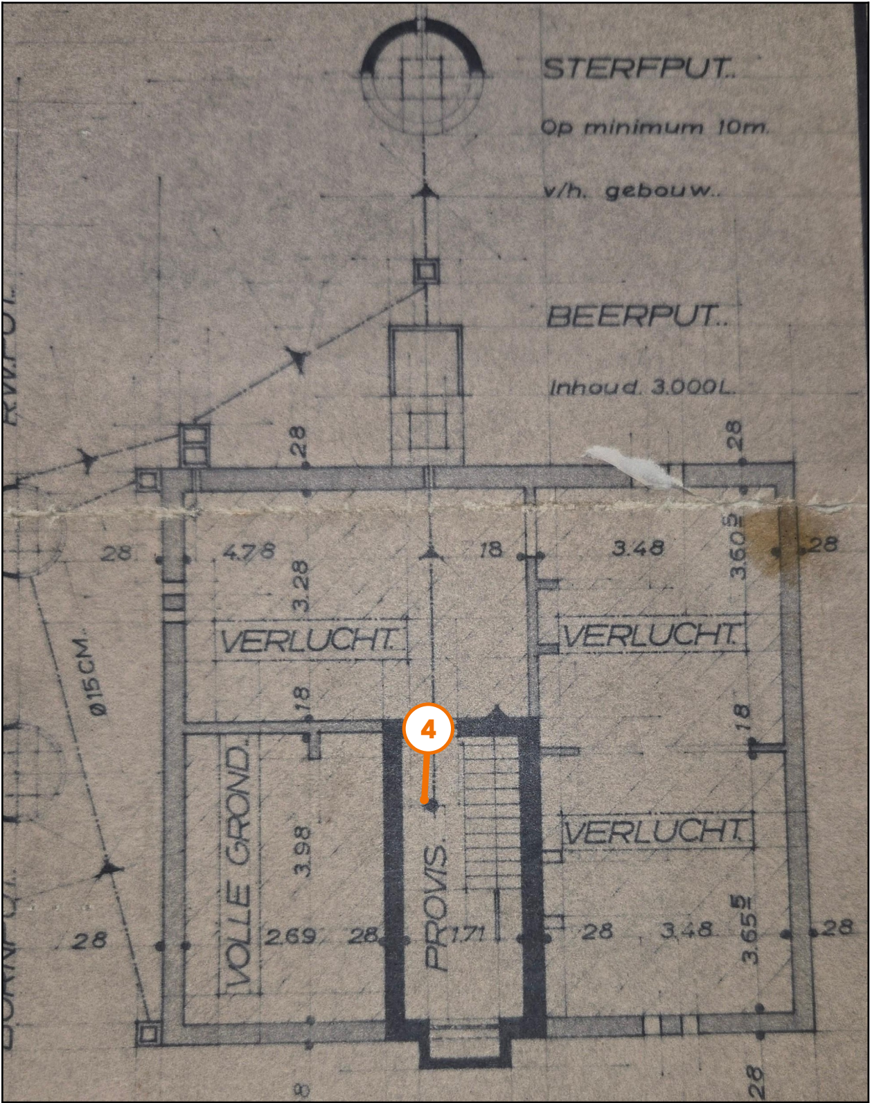
Legende van plan 1.1: Plan kelder
