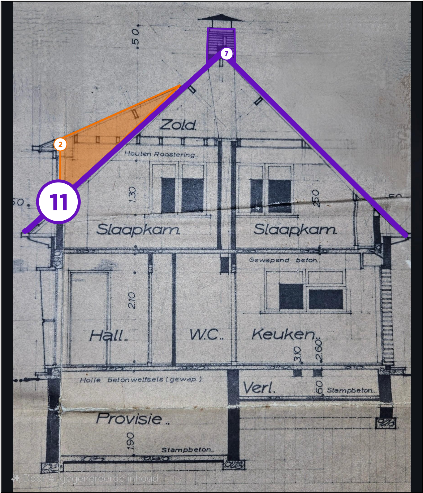
Legende van plan 1.4: Plan doorsnede
