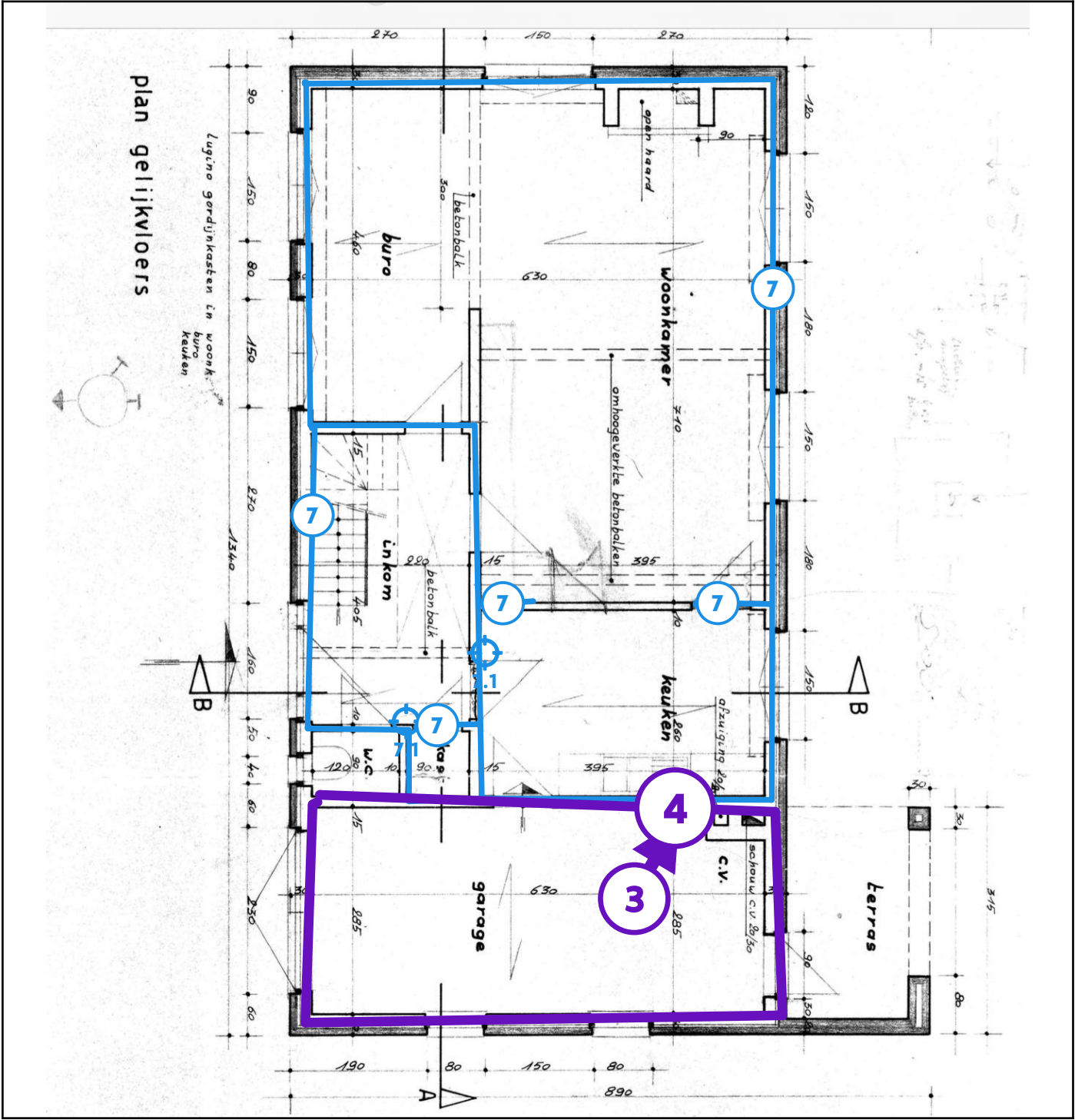
Legende van plan 1.1: Grondplan glv
