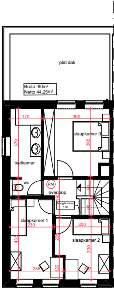
1e verdieping
