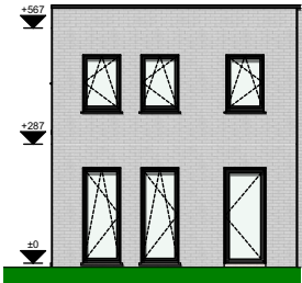
Voorgevel
