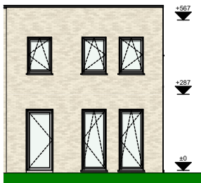
Voorgevel
