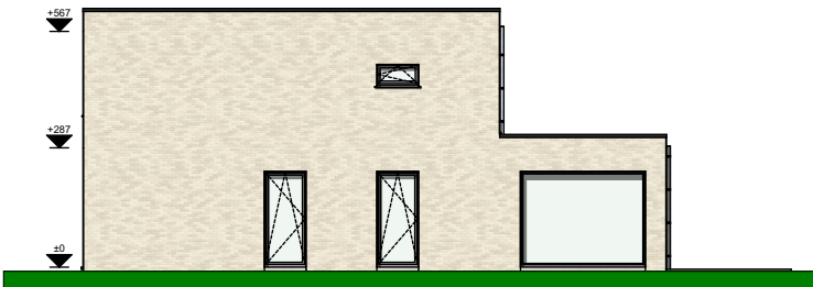
Rechtergevel
