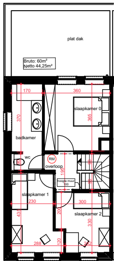
1e verdieping
