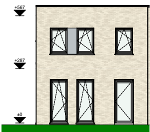
Voorgevel
