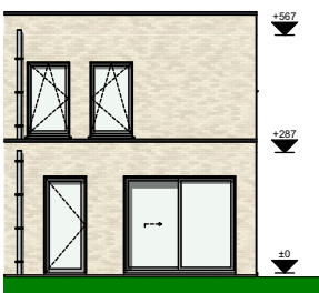
Achtergevel
