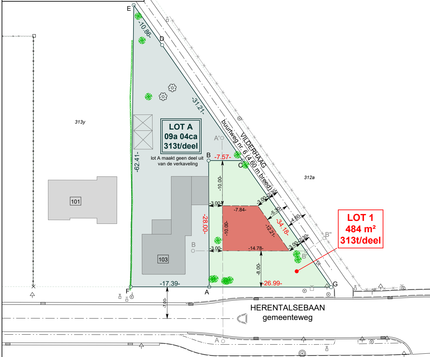
VERKAVELINGSPLAN NIEUWE TOESTAND
