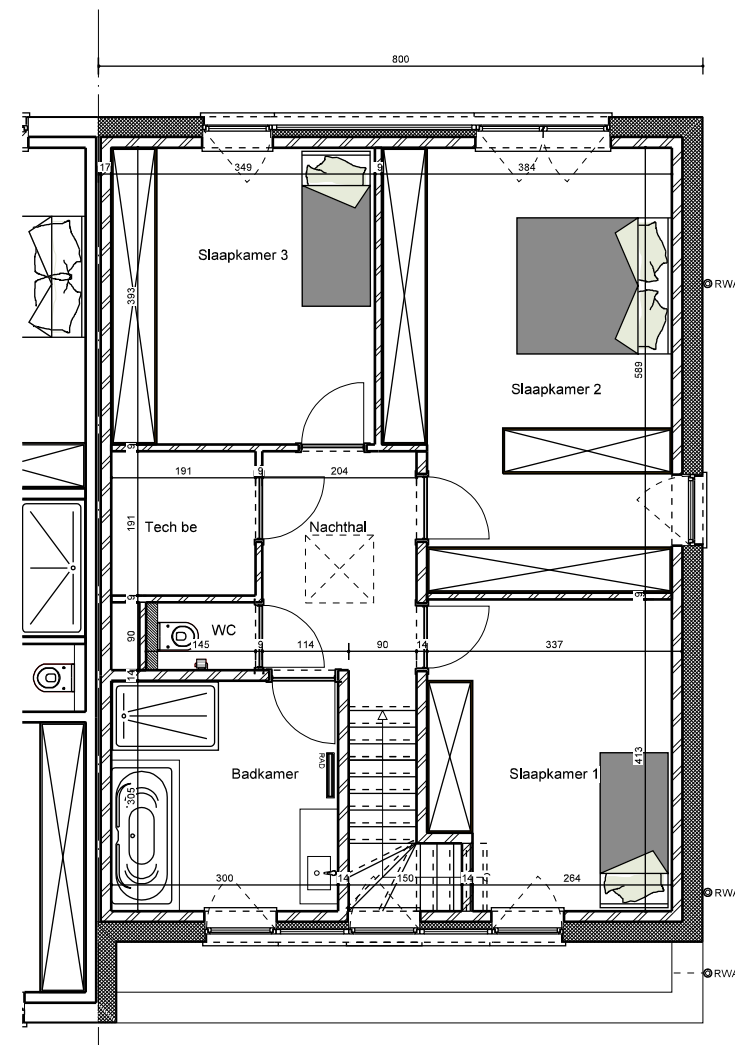
Verdieping
