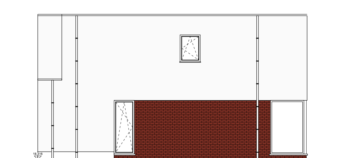
Zijgevel
