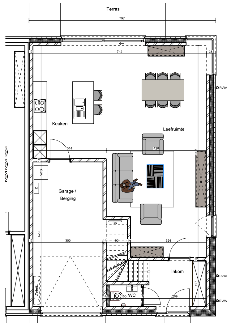
Begane grond
