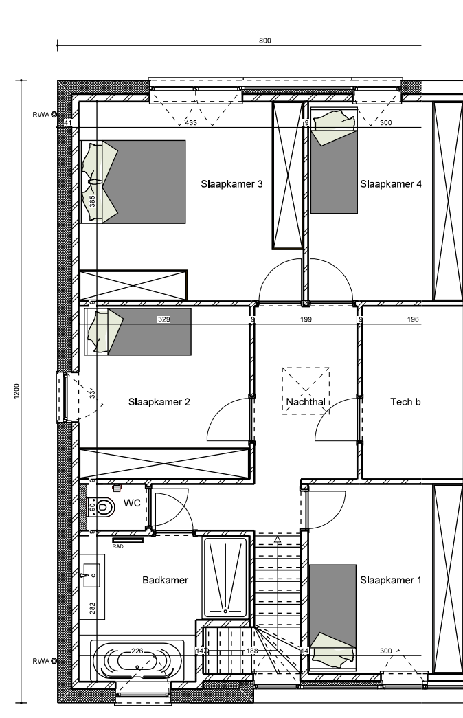
Verdieping
