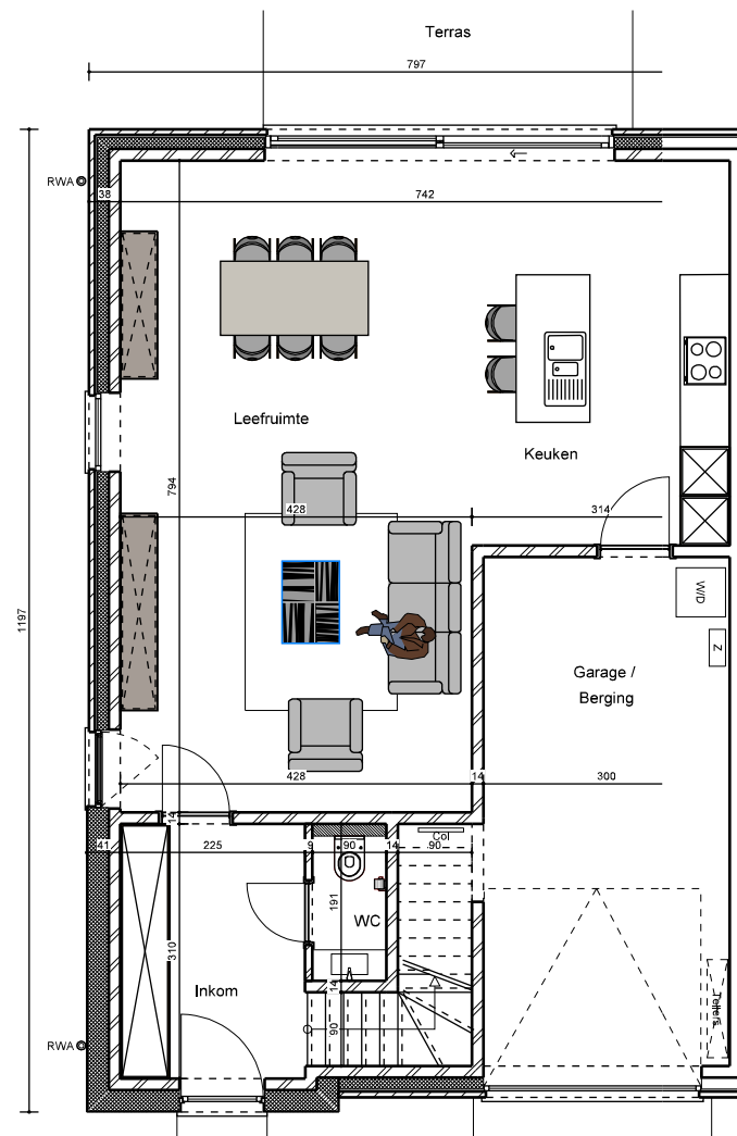
Begane grond
