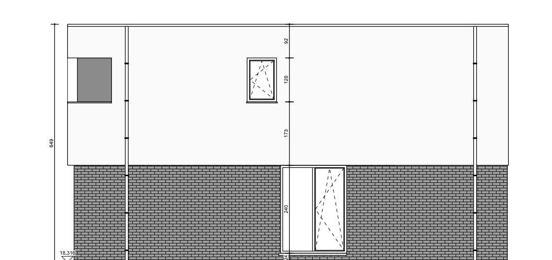
Zijgevel
