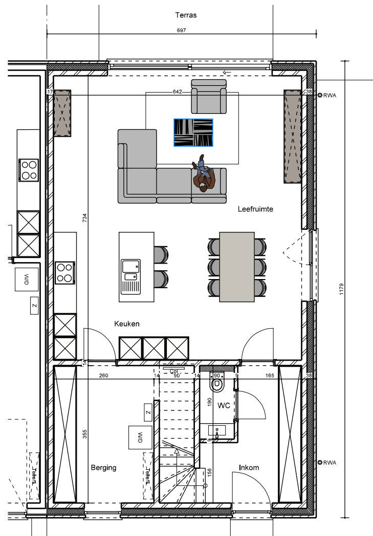
Begane grond
