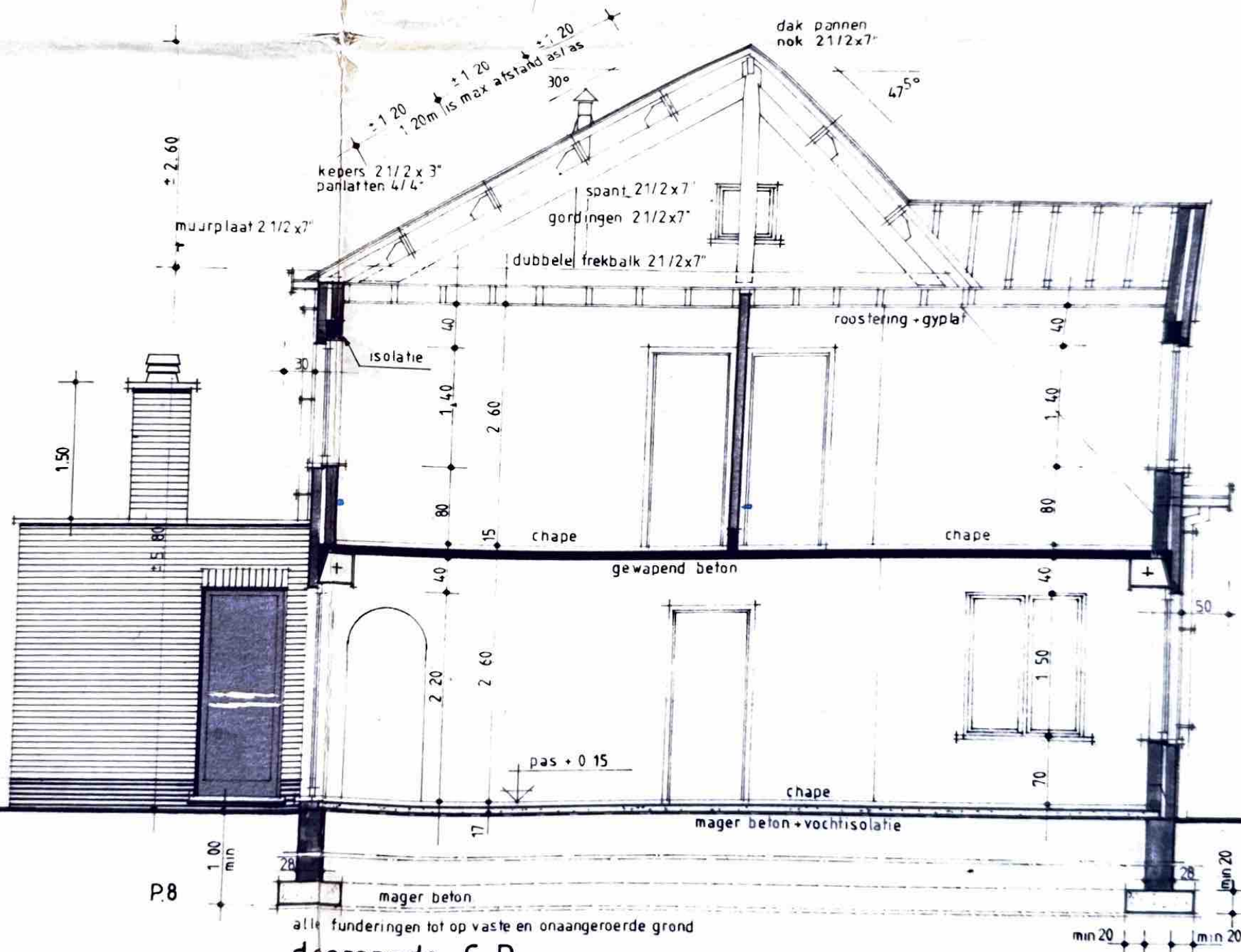
doorsnede C. D.
